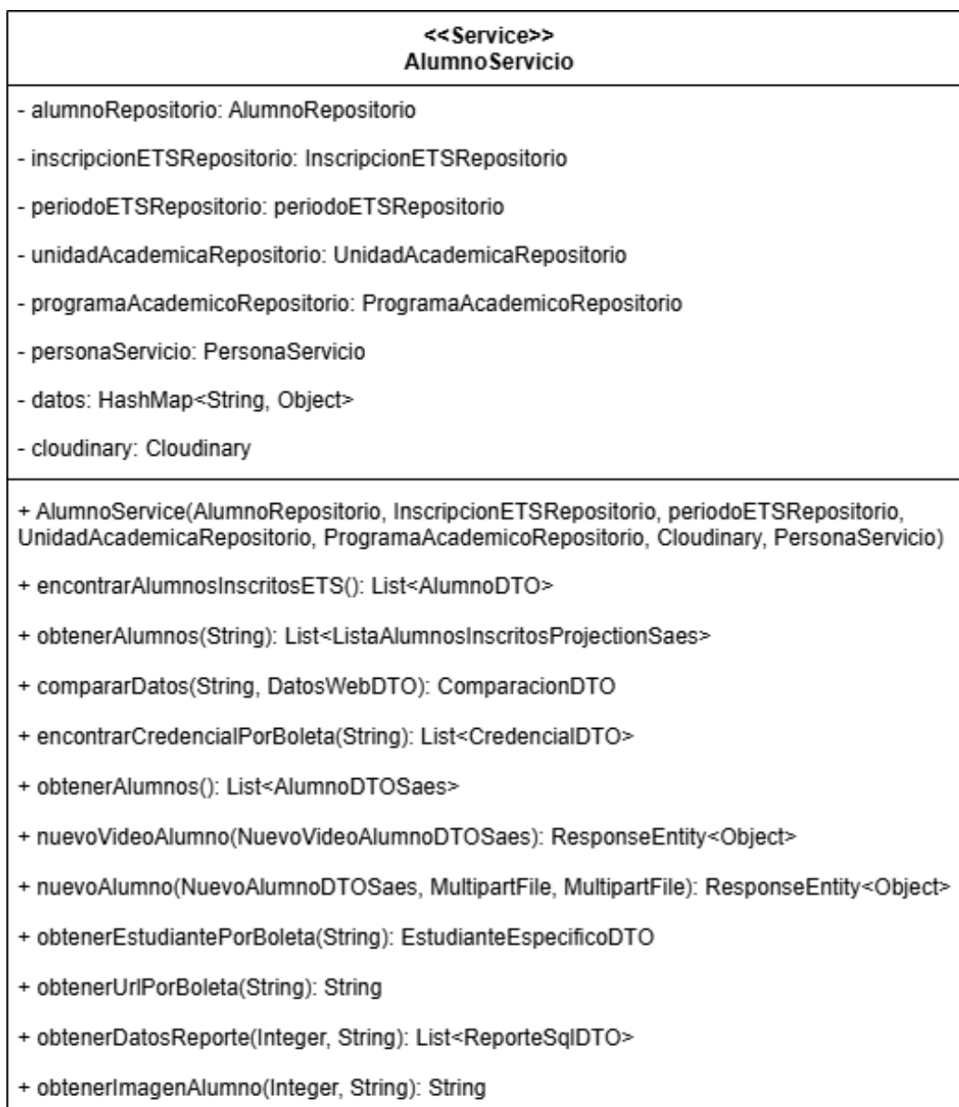
Figura B.12: Diagrama de clase AlumnoServicio de los servicios del servidor parte 1.
