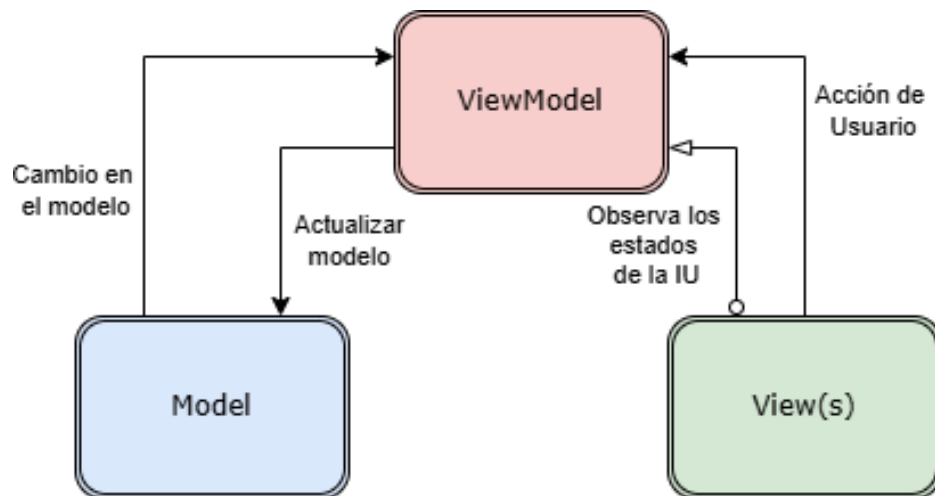
Figura 5.1: Arquitectura MVVM.
