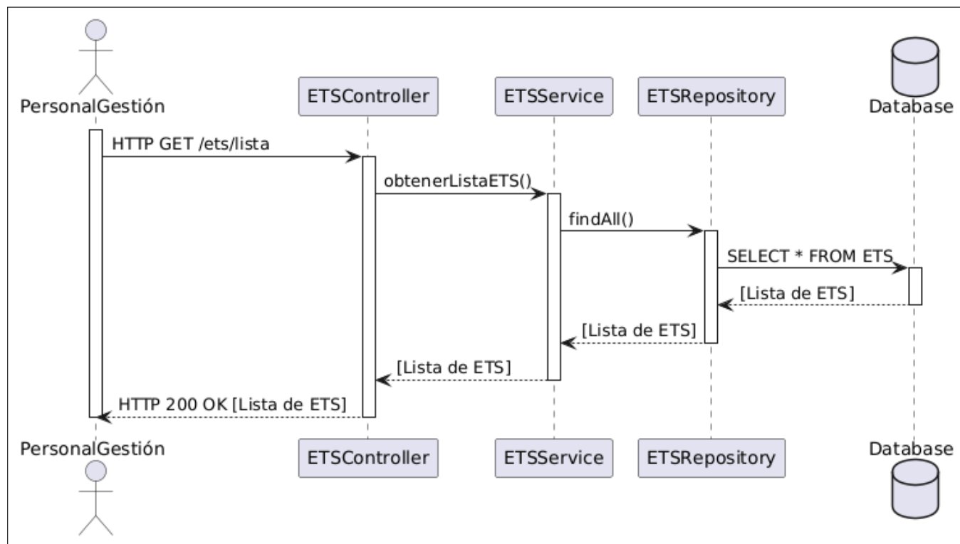
Figura B.87: Diagrama de secuencia del caso de uso número 28 (Consultar lista de ETS).
