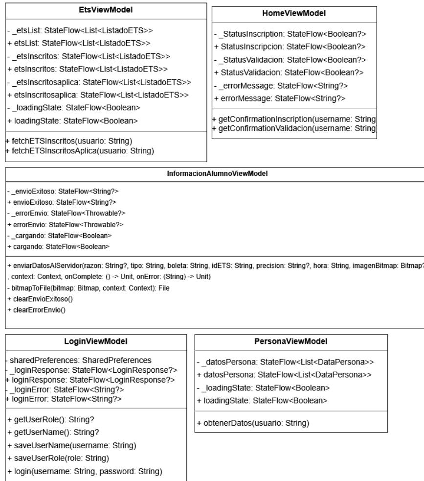
Figura B.54: Diagrama de clases para package.example.prueba3.Views parte 2.
