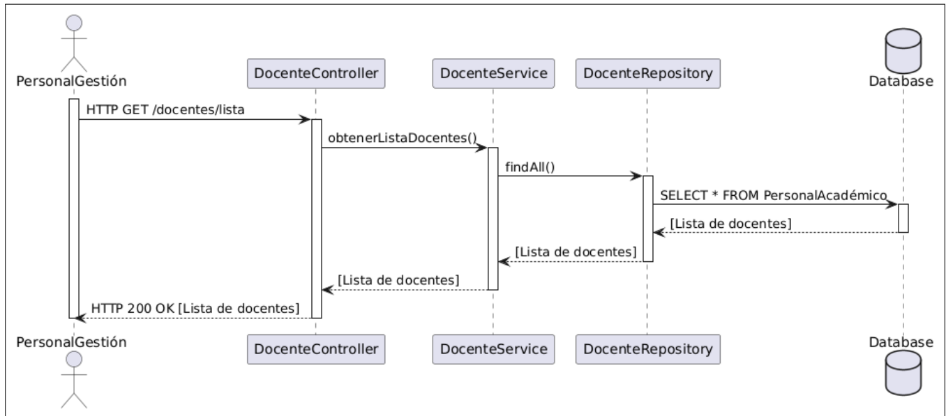
Figura B.91: Diagrama de secuencia del caso de uso número 36 (Consultar lista de docentes).
