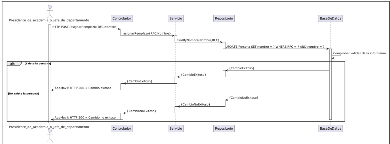
Figura B.95: Diagrama de secuencia del caso de uso número 42 (Asignar docente de remplazo).
