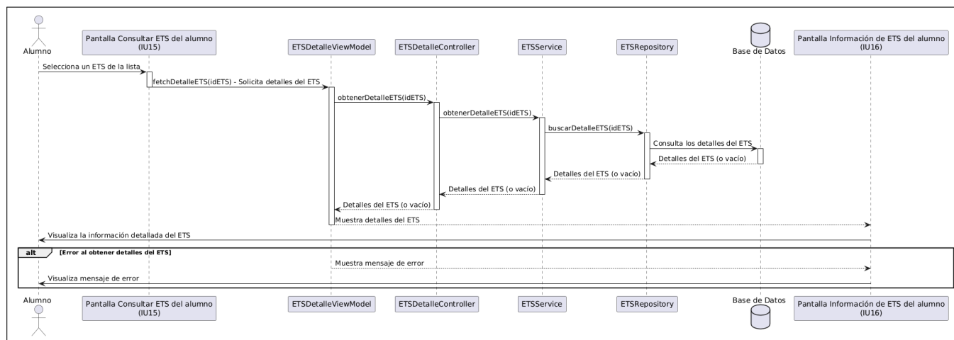
Figura B.80: Diagrama de secuencia del caso de uso número 18 (Mostrar información del los ETS inscritos).
