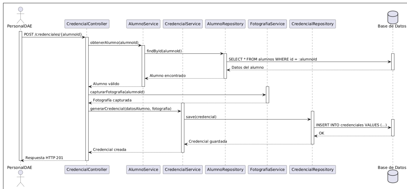
Figura B.84: Diagrama de secuencia del caso de uso número 22 y 23 (Crear credencial y capturar fotografía estudiantil).
