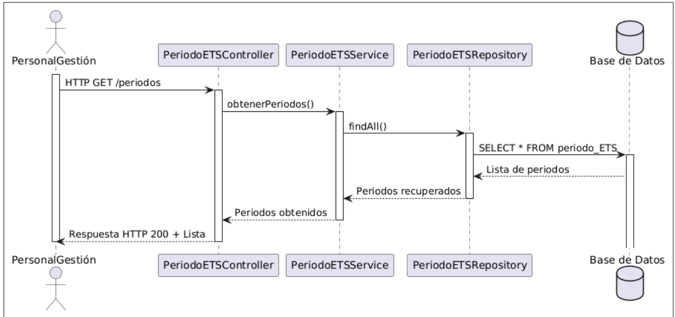
Figura B.85: Diagrama de secuencia del caso de uso número 24 (Consultar lista de periodo de ETS).
