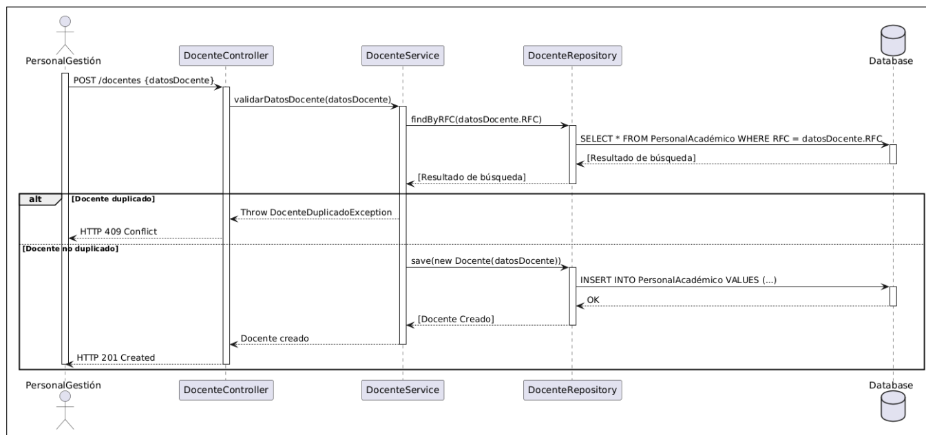
Figura B.92: Diagrama de secuencia del caso de uso número 37 (Dar de alta docente).
