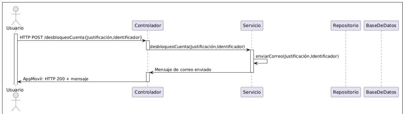
Figura B.93: Diagrama de secuencia del caso de uso número 40 (Solicitar desbloqueo de cuenta).
