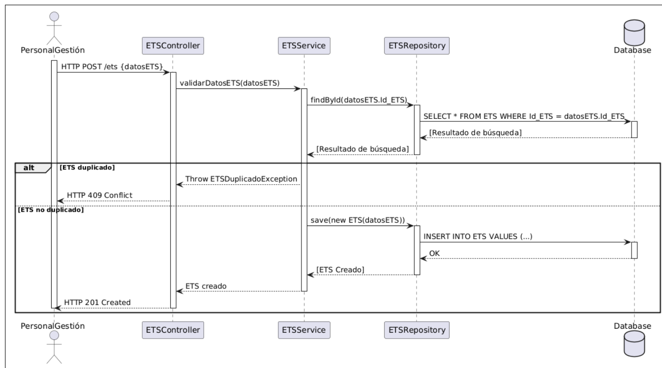
Figura B.88: Diagrama de secuencia del caso de uso número 29 (Dar de alta ETS).
