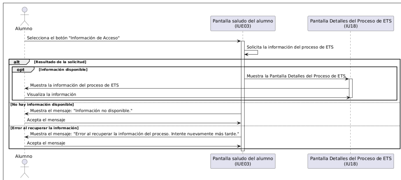
Figura B.82: Diagrama de secuencia del caso de uso número 20 (Revisar información de acceso a los ETS).
