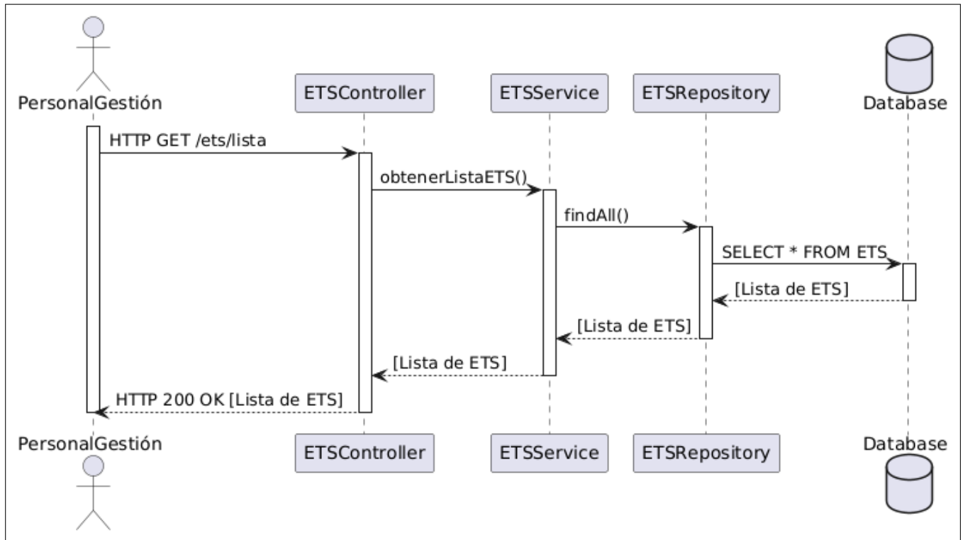
Figura B.87: Diagrama de secuencia del caso de uso número 28 (Consultar lista de ETS).
