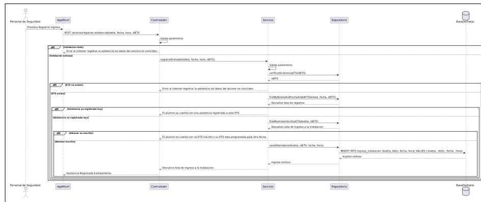
Figura B.77: Diagrama de secuencia del caso de uso número 15 (Registrar asistencia).
