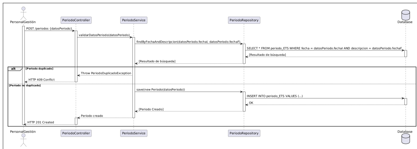
Figura B.86: Diagrama de secuencia del caso de uso número 25 (Dar de alta de periodo de ETS).
