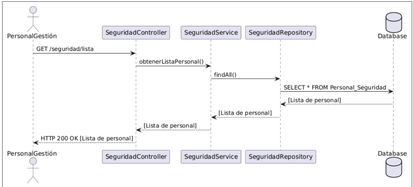
Figura B.89: Diagrama de secuencia del caso de uso número 32 (Consultar lista de personal de seguridad).
