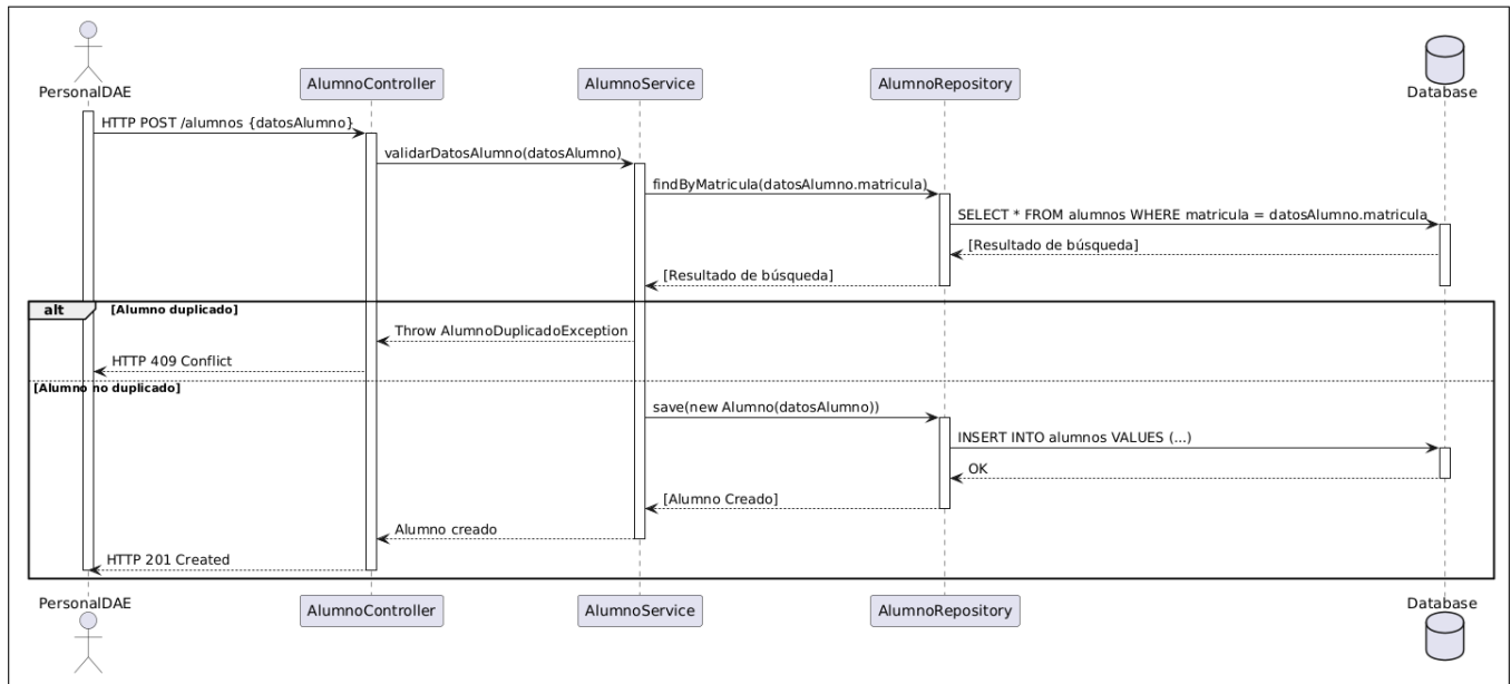
Figura B.83: Diagrama de secuencia del caso de uso número 21 (Dar de alta a alumno).
