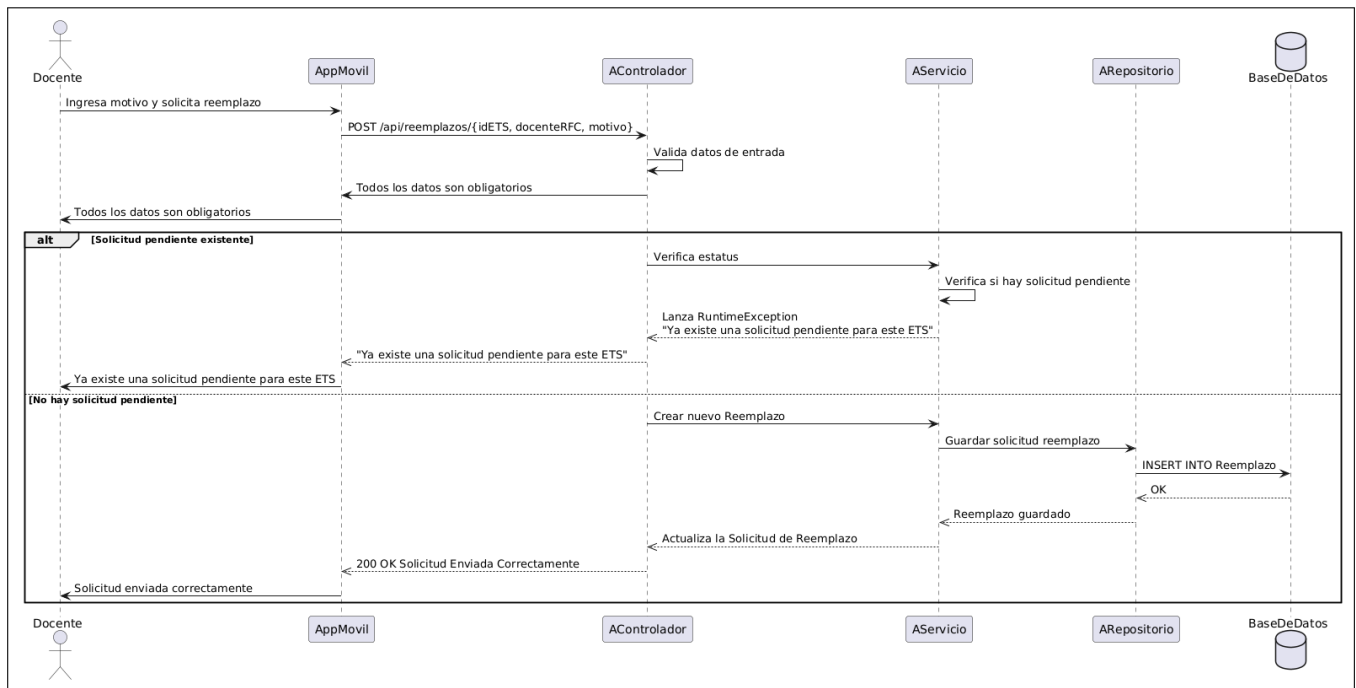
Figura B.69: Diagrama de secuencia del caso de uso número 07 (Solicitar reemplazo).
