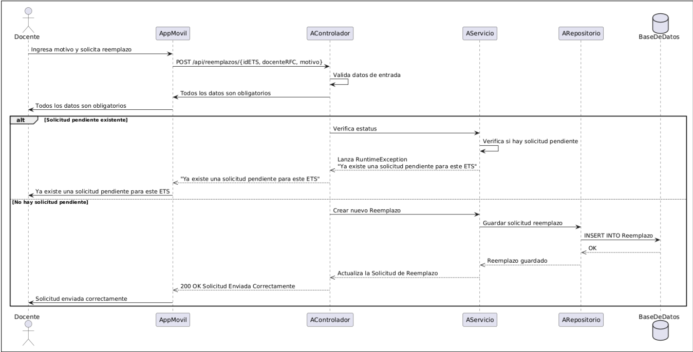
Figura B.70: Diagrama de secuencia del caso de uso número 07 (Solicitar remplazo).
