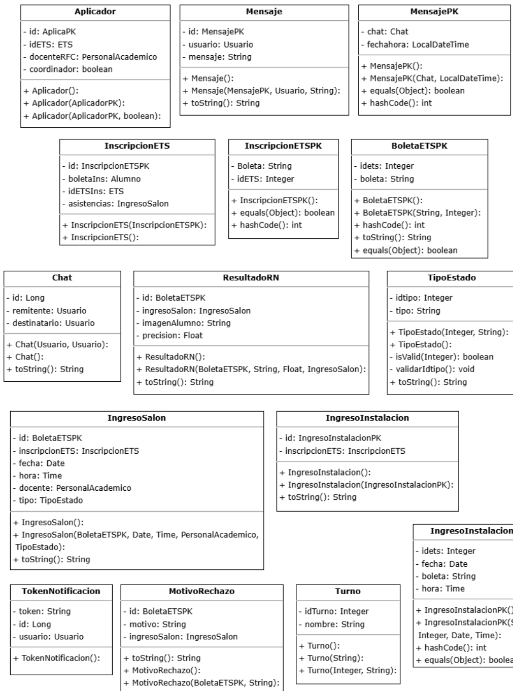
Figura 5.6: Diagrama de clases de las entidades del servidor parte 3.
