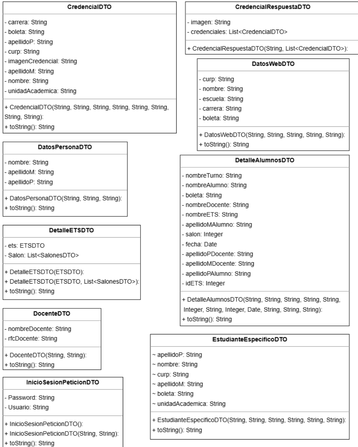
Figura 5.25: Diagrama de clases de los DTO del servidor parte 4.
