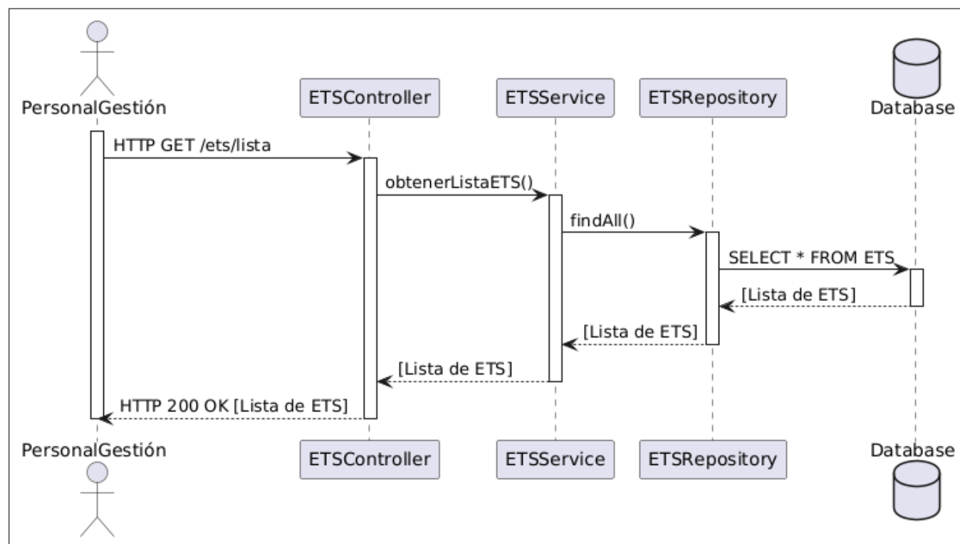
Figura 5.87: Diagrama de secuencia del caso de uso número 28 (Consultar lista de ETS).
