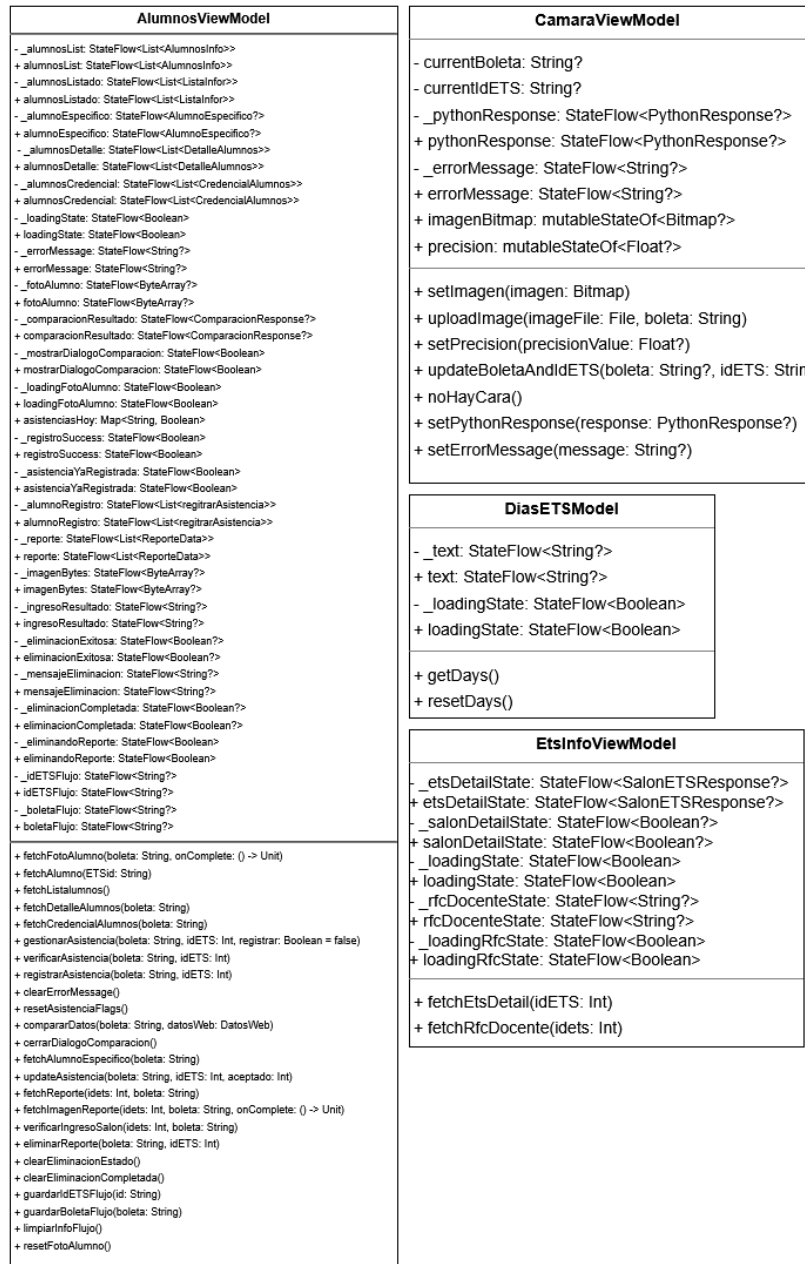
Figura 5.53: Diagrama de clases para package.example.prueba3.Views parte 1.
