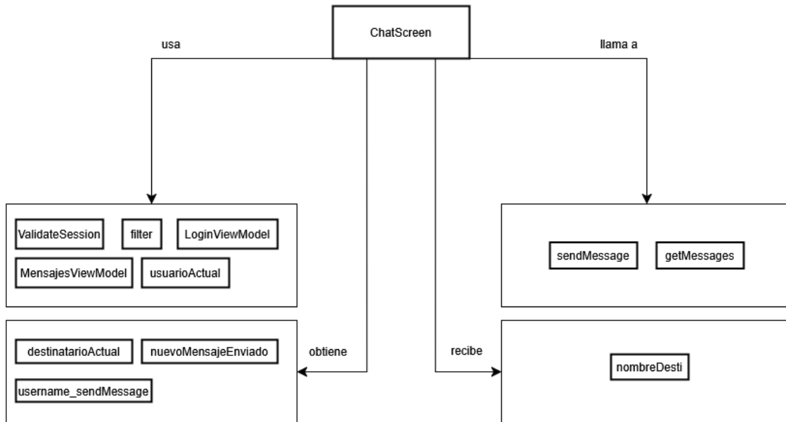
Figura 5.32: Diagrama de componentes para ChatScreen.kt .
