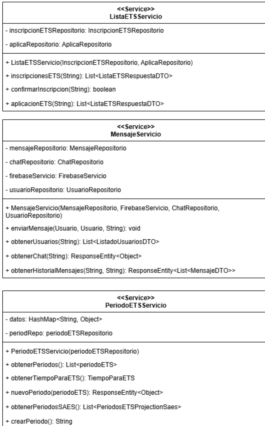
Figura 5.15: Diagrama de clases de los servicios del servidor parte 4.
