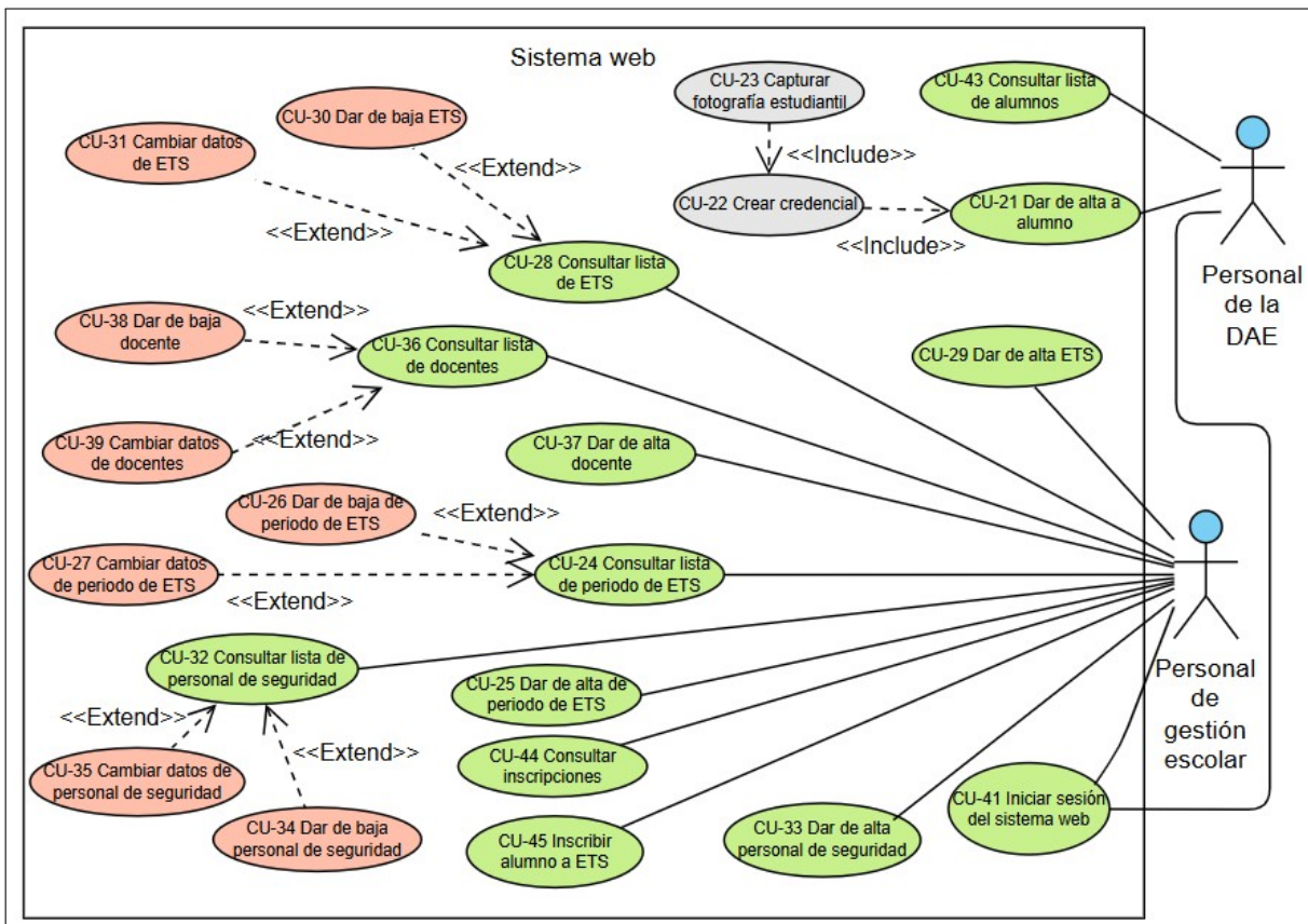
Figura 4.6: Diagrama de casos de uso del sistema web.
