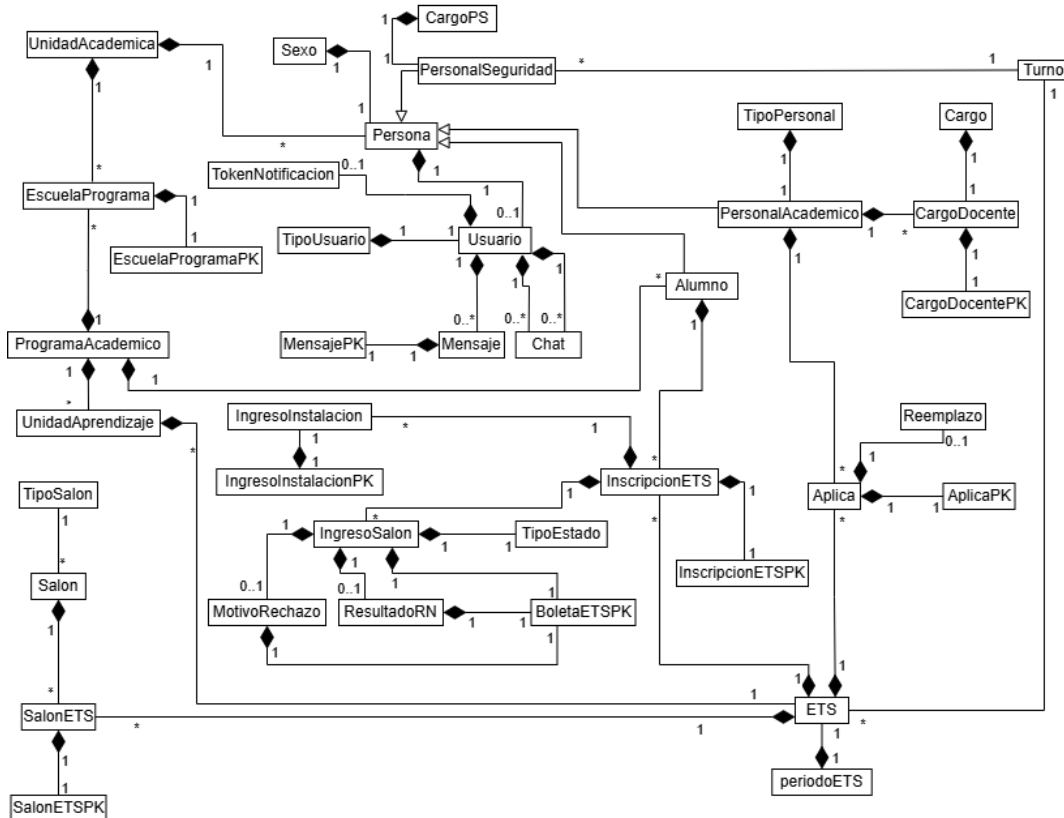
Figura 5.3: Diagrama de clases general de las entidades del servidor.
