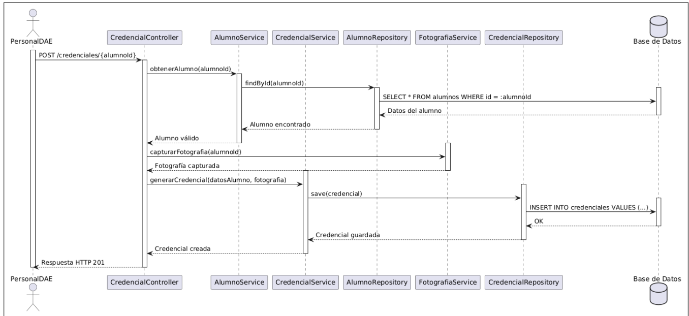
Figura 5.84: Diagrama de secuencia del caso de uso número 22 y 23 (Crear credencial y capturar fotografía estudiantil).
