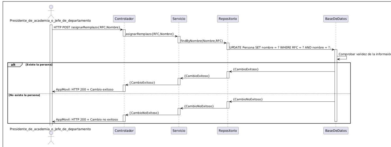
Figura B.83: Diagrama de secuencia del caso de uso número 42 (Asignar docente de replazo).
