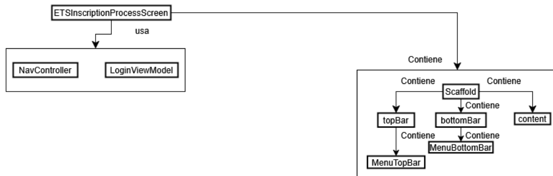
Figura B.37: Diagrama de componentes para EtsInscriptionProcessScreen.kt .
