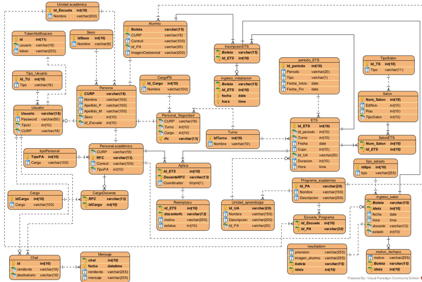
Figura A.1: Modelo del dominio del problema
