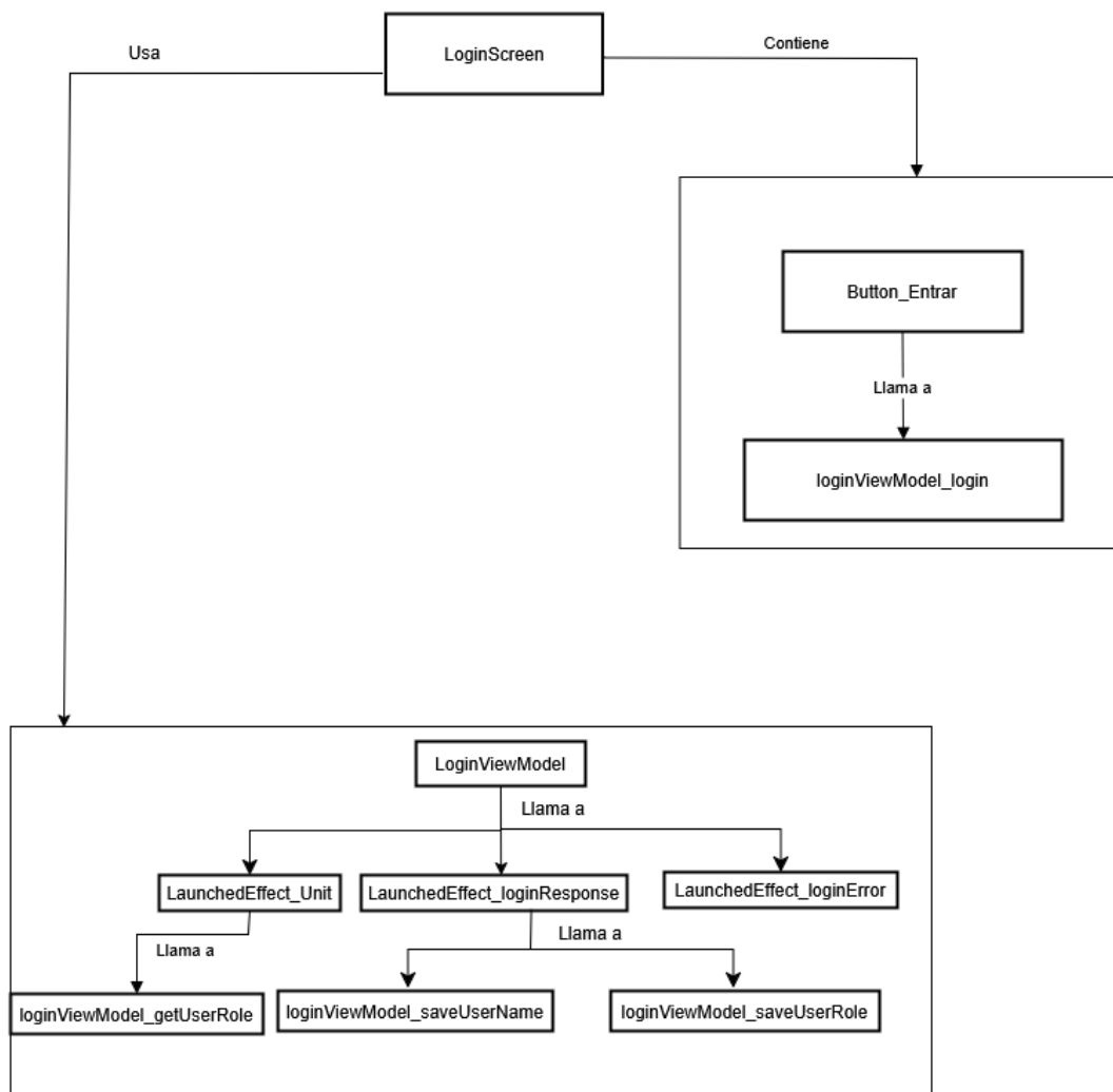
Figura 5.43: Diagrama de componentes para LoginScreen.kt .
