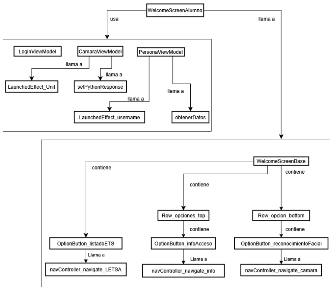
Figura 5.51: Diagrama de componentes para WelcomeScreenAlumno.kt .
