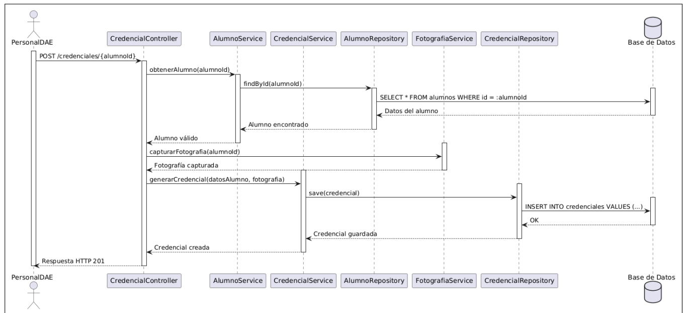
Figura B.84: Diagrama de secuencia del caso de uso número 22 y 23 (Crear credencial y capturar fotografía estudiantil).
