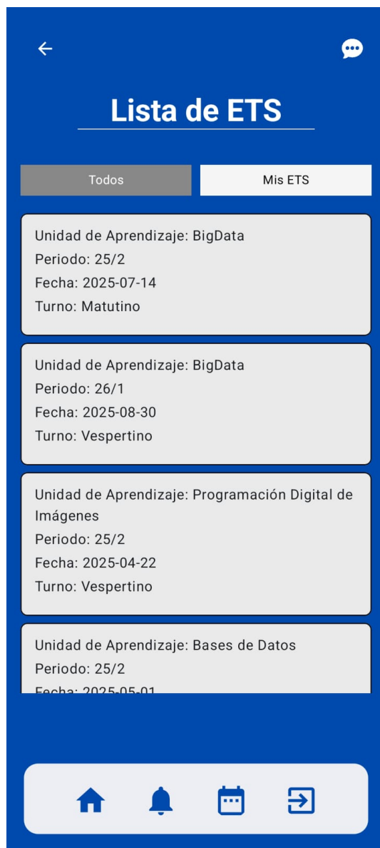
Figura A.13: IU05 Pantalla Consultar ETS.
