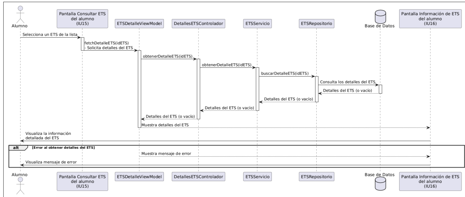
Figura B.80: Diagrama de secuencia del caso de uso número 18 (Mostrar información de los ETS inscritos).
