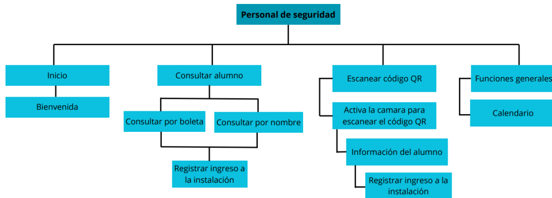
Figura 4.10: Mapa de navegación del personal de seguridad
