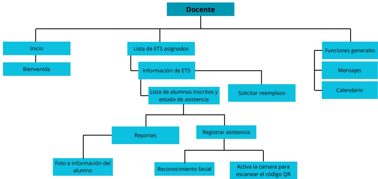
Figura 4.9: Mapa de navegación del docente
