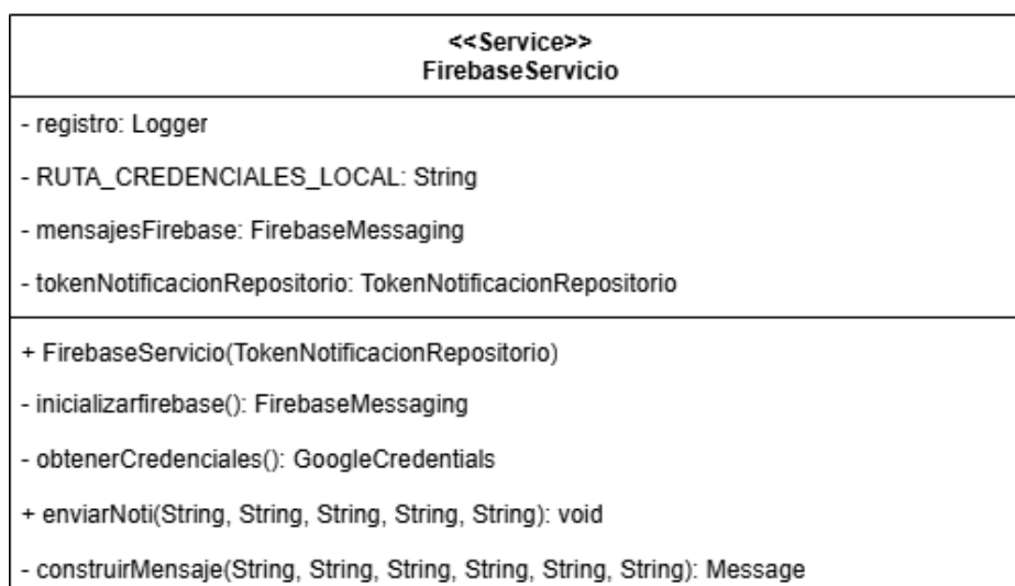
Figura A.13: Diagrama de clases de los servicios del servidor parte 2.
