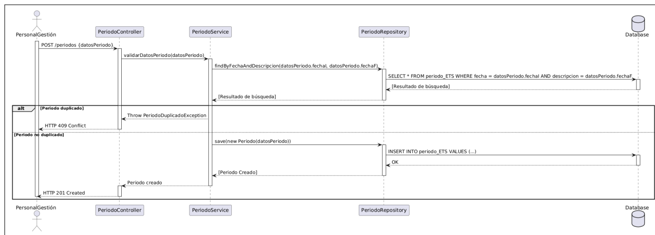
Figura B.86: Diagrama de secuencia del caso de uso número 25 (Dar de alta de periodo de ETS).
