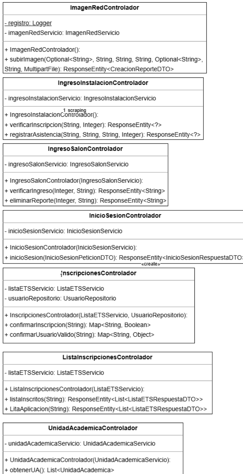
Figura 5.9: Diagrama de clases de los controladores del servidor parte 3.
