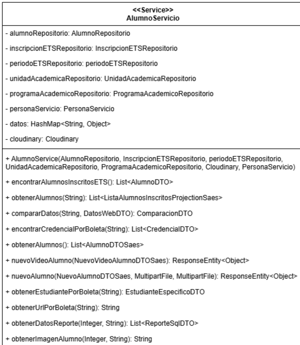
Figura 5.12: Diagrama de clases de los servicios del servidor parte 1.
