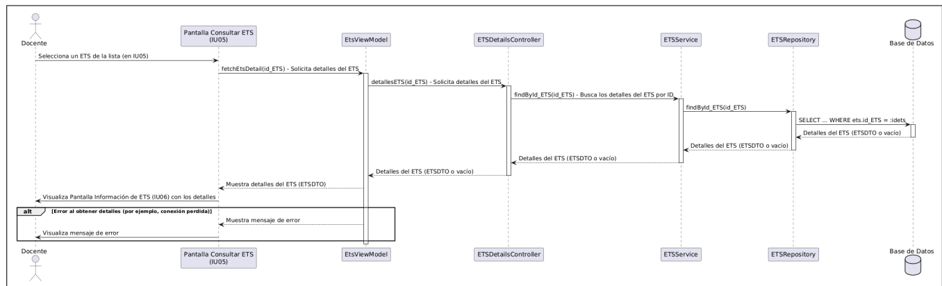
Figura 5.68: Diagrama de secuencia del caso de uso número 06 (Mostrar información de los ETS asignados).
