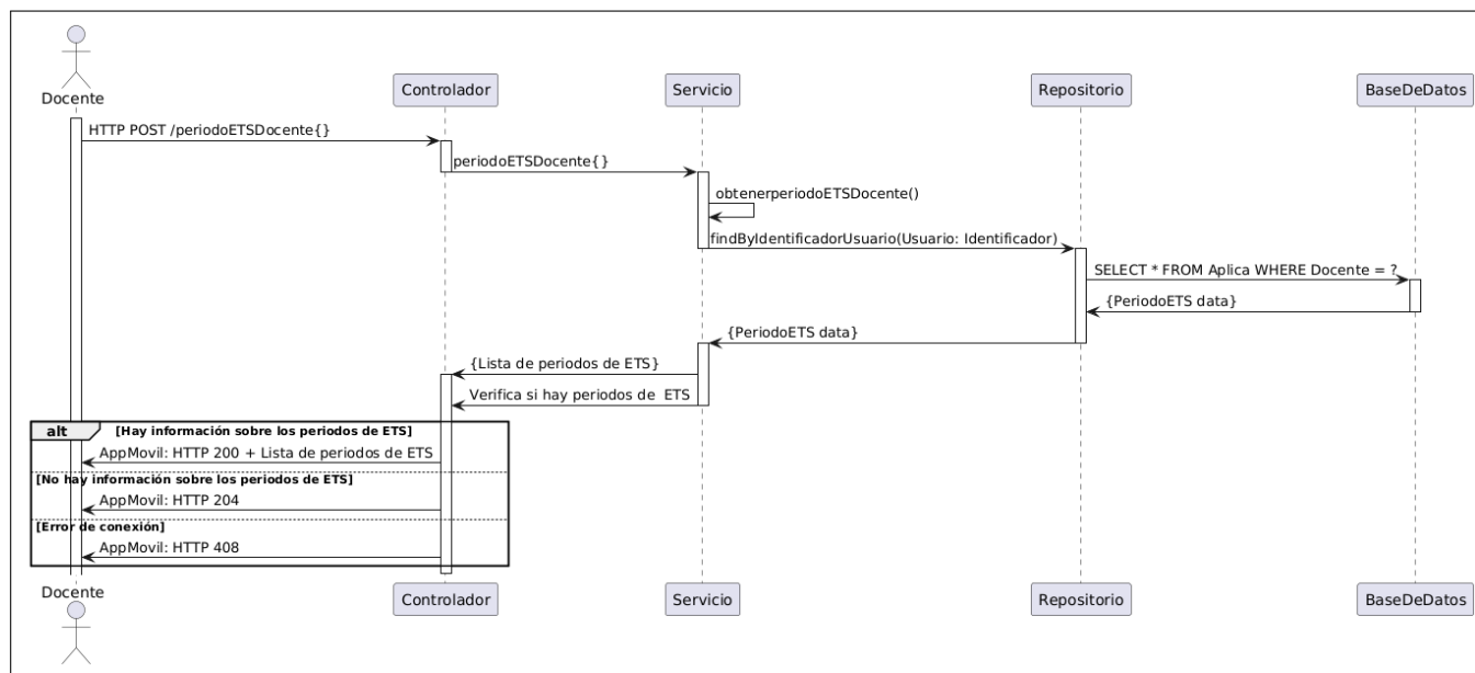
Figura 5.66: Diagrama de secuencia del caso de uso número 04 (Consultar periodos de ETS asignados al docente).
