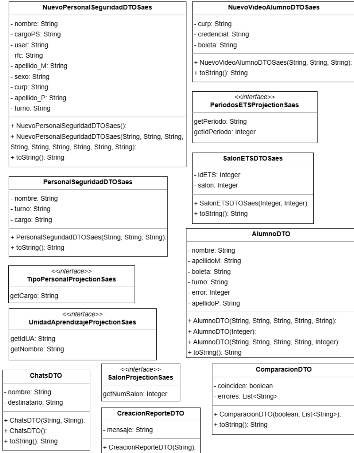
Figura 5.24: Diagrama de clases de los DTO del servidor parte 3.
