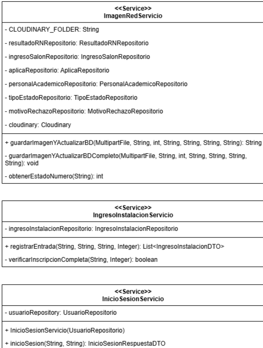
Figura 5.14: Diagrama de clases de los servicios del servidor parte 3.
