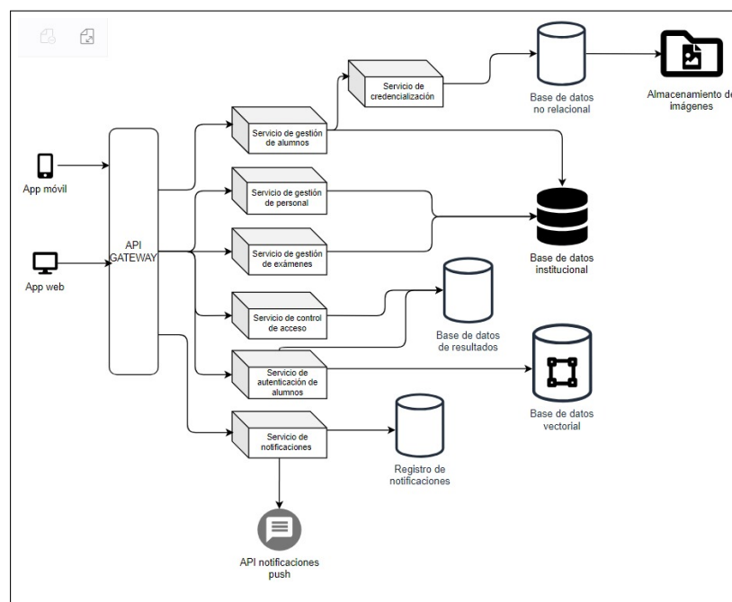
Figura 4.1: Arquitectura del sistema.
