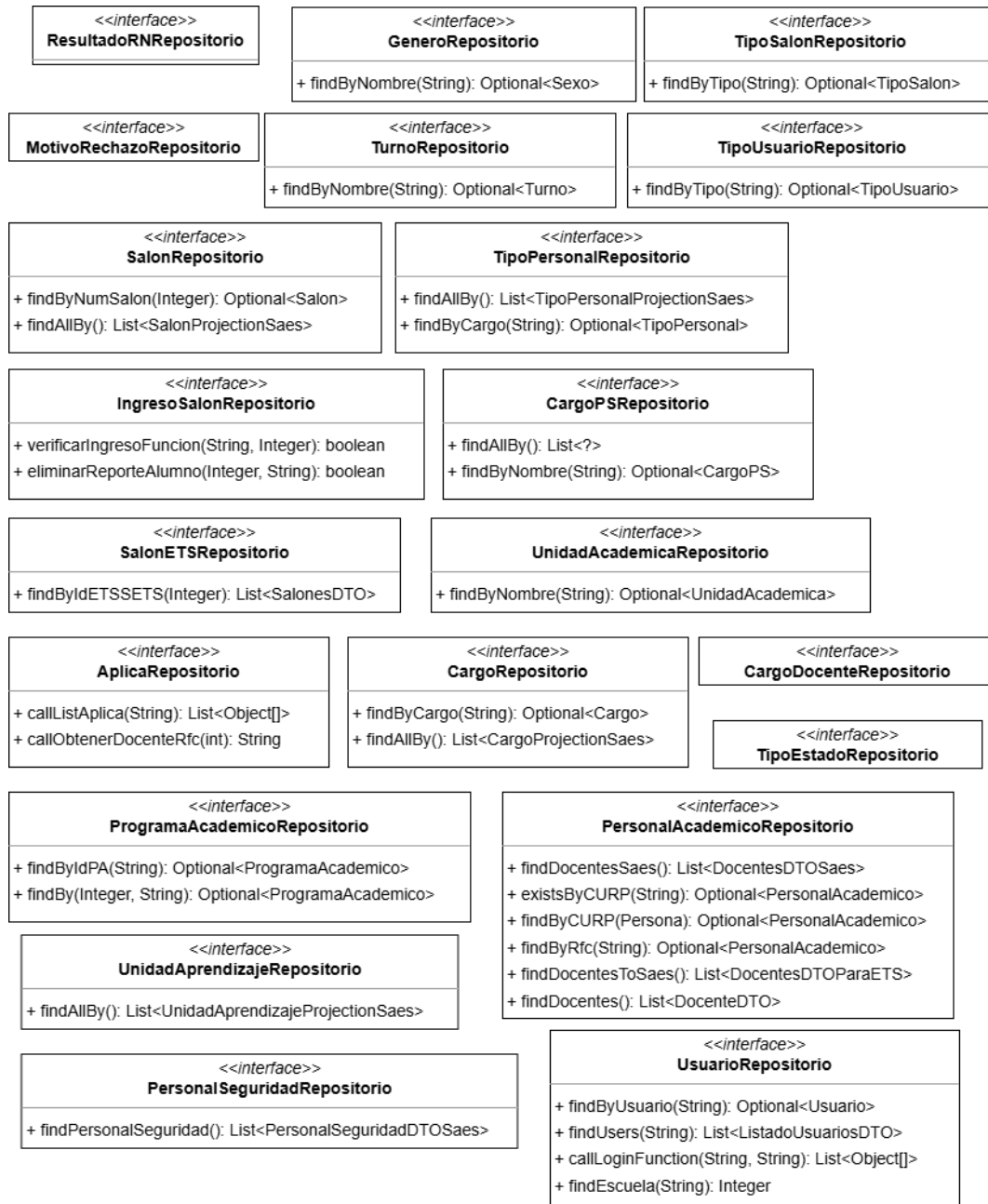
Figura 5.20: Diagrama de clases de los repositorios del servidor parte 1.
