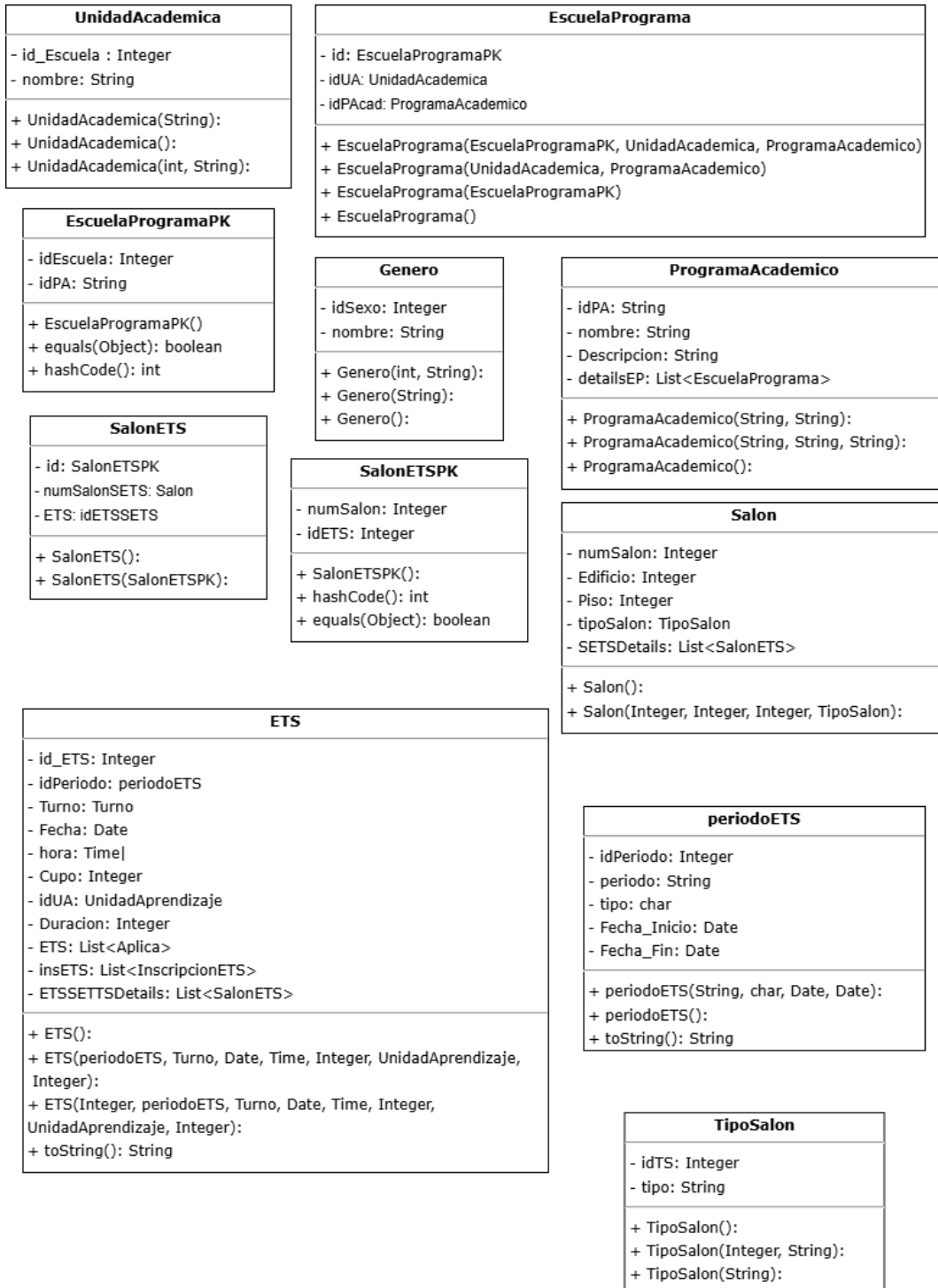
Figura 5.4: Diagrama de clases de las entidades del servidor parte 1.
