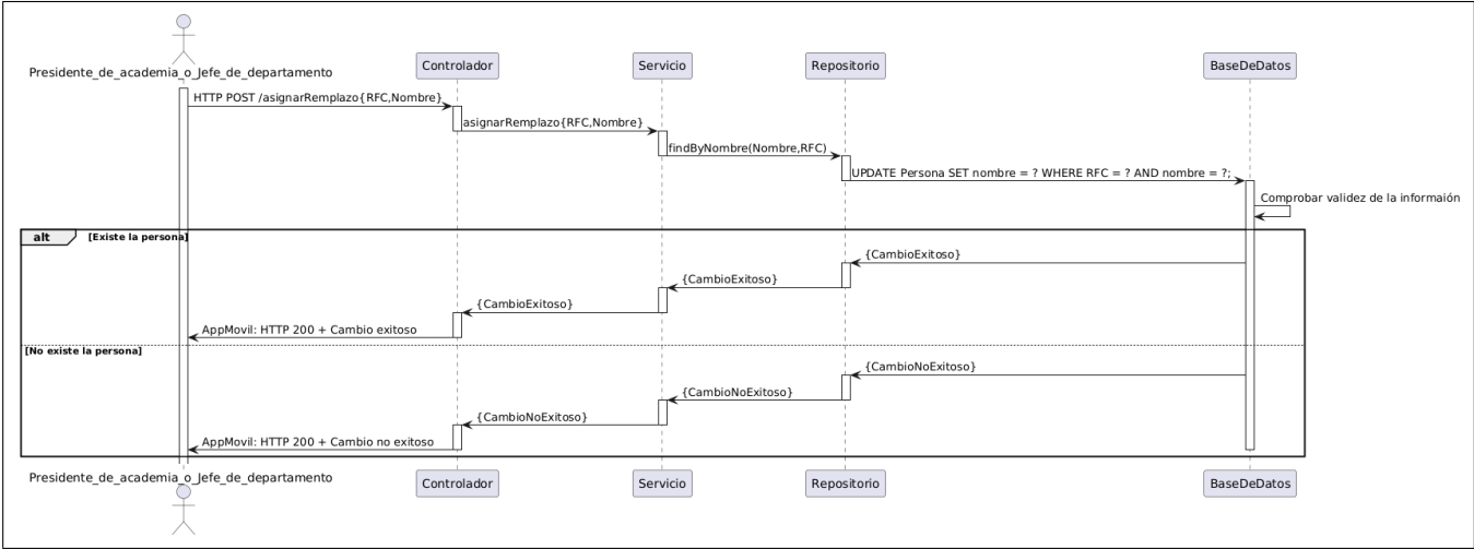
Figura A.84: Diagrama de secuencia del caso de uso número 42 (Asignar docente de replazo).
