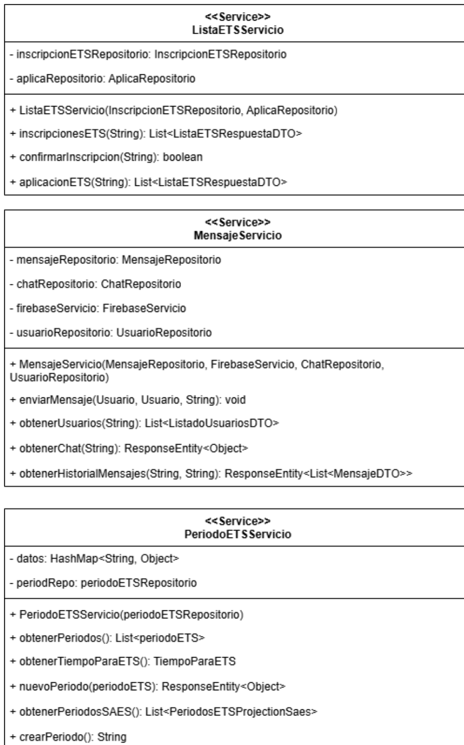
Figura A.15: Diagrama de clases de los servicios del servidor parte 4.
