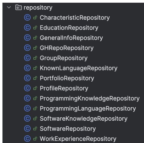
Abbildung 61: Repository - Klassen
