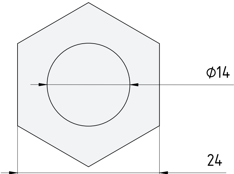
Nut Dimensions
