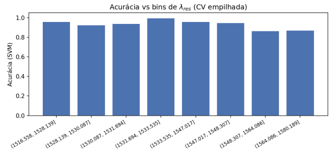
Figura 3. Acurácia do SVM por bin de \lambda_{res} (CV empilhada).
