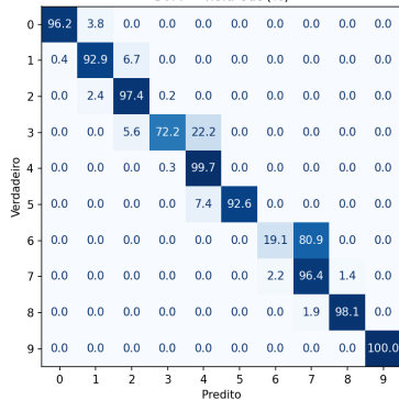
SVM
