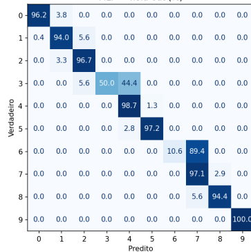
MLP
