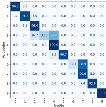
kNN
