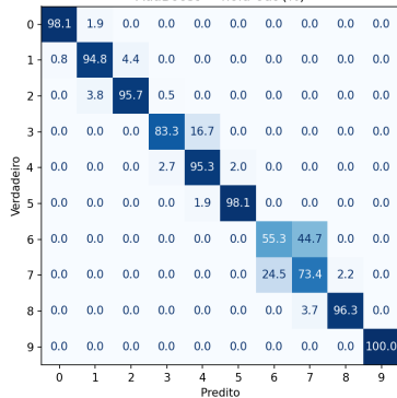
AdaBoost
