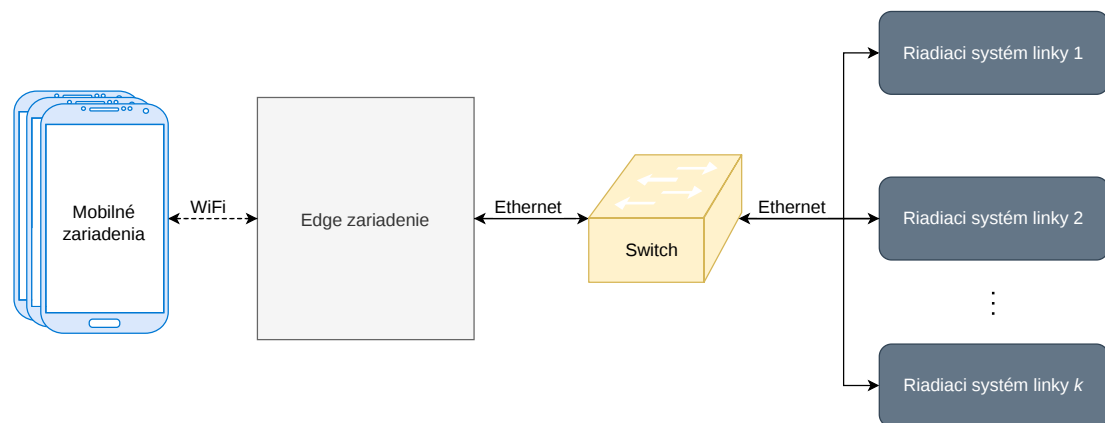
Obr. 4: Fyzická topológia systému
