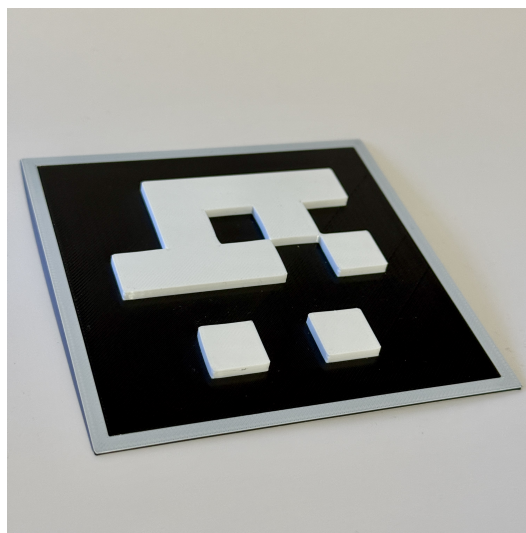
Obr. 5: ArUco marker tlačený z vygenerovaného STL modelu
