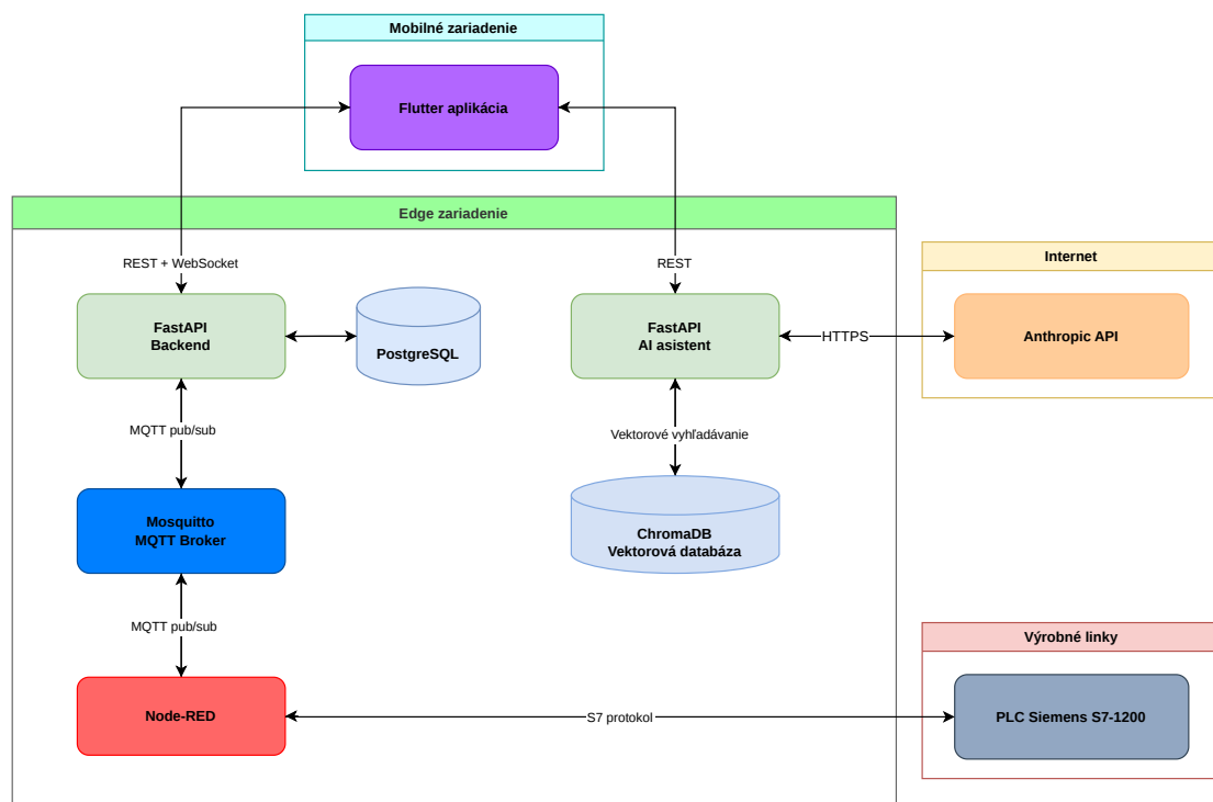
Obr. 3: Diagram architektúry systému a komunikácia medzi komponentmi
