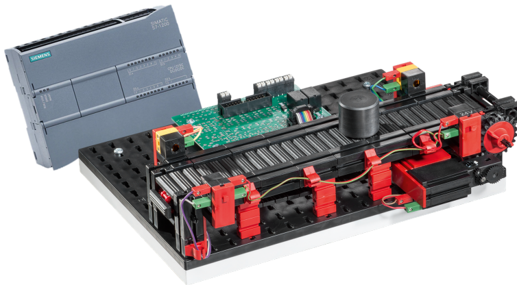
Obr. 19: Model dopravníka Fischertechnik a PLC Siemens S7-1200
