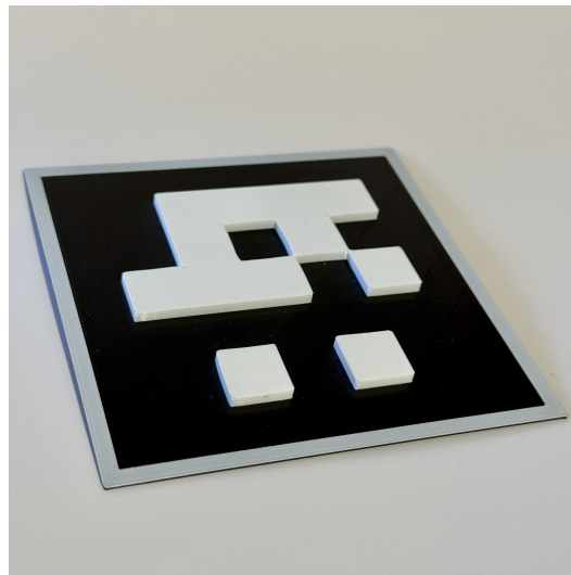
Obr. 7: ArUco marker tlačený z vygenerovaného STL modelu
