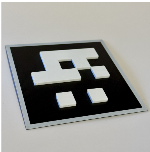
Obr. 7: ArUco marker tlačný z vygenerovaného STL modelu
