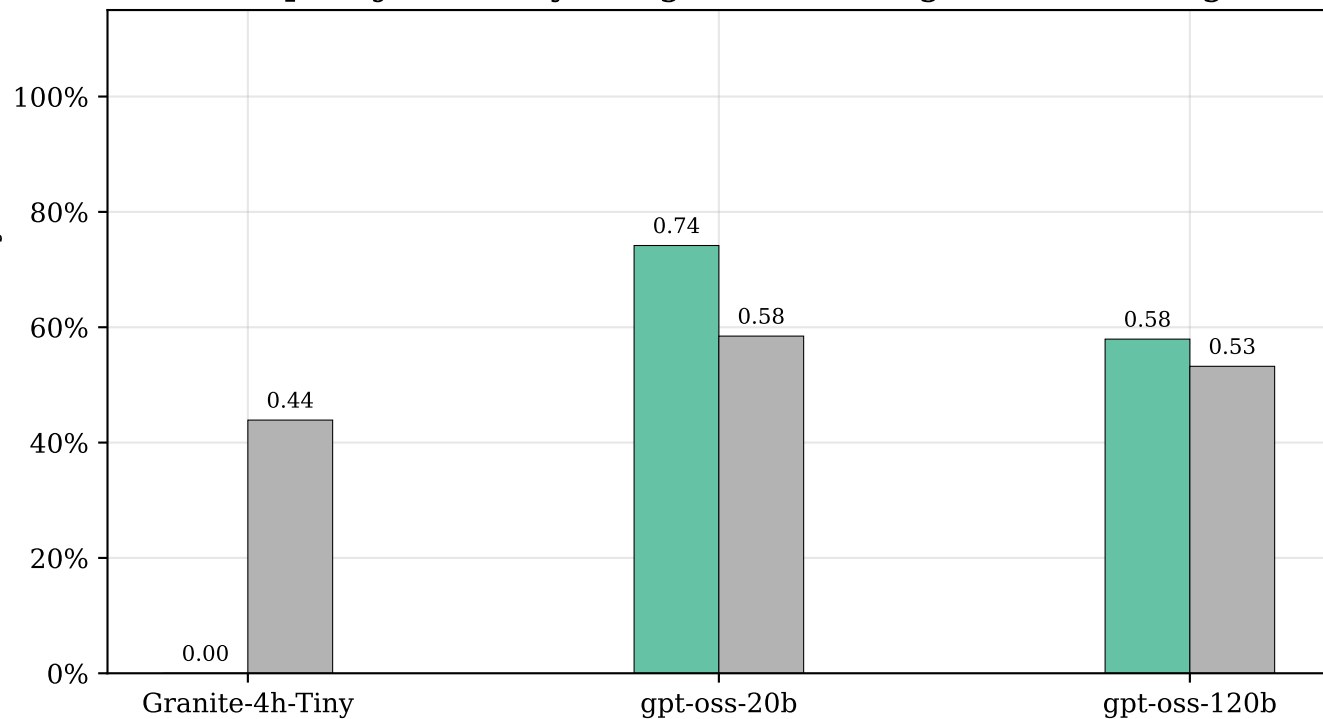
Porównanie miary precyzji dla wybranych dużych modeli językowych oraz podejścia klasycznego i autorskiego łańcuchowego
