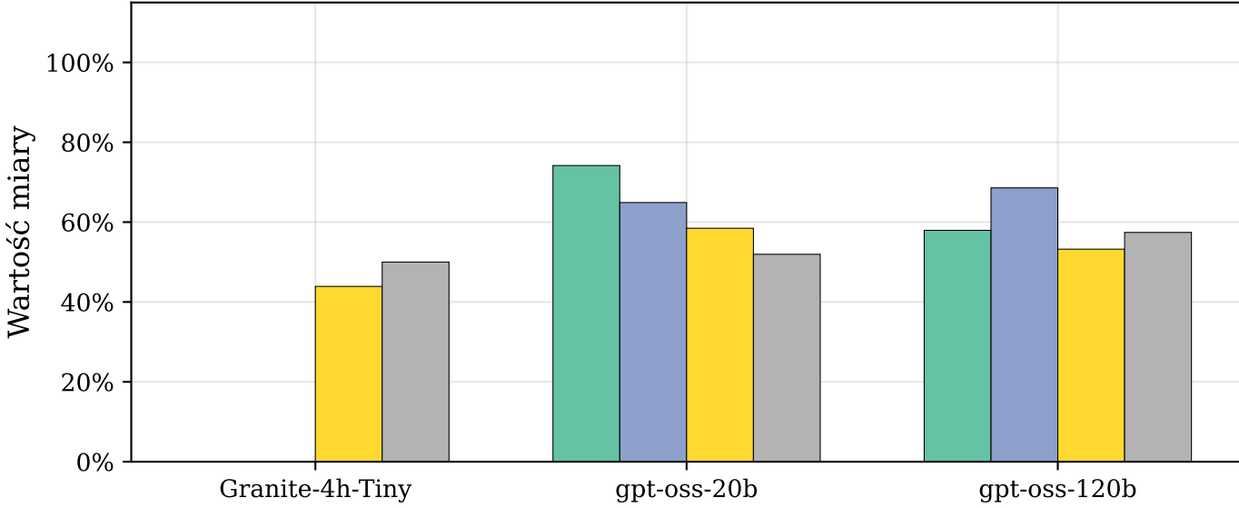
Porównanie miary F1 dla wybranych dużych modeli językowych oraz podejścia klasycznego i autorskiego łańcuchowego
