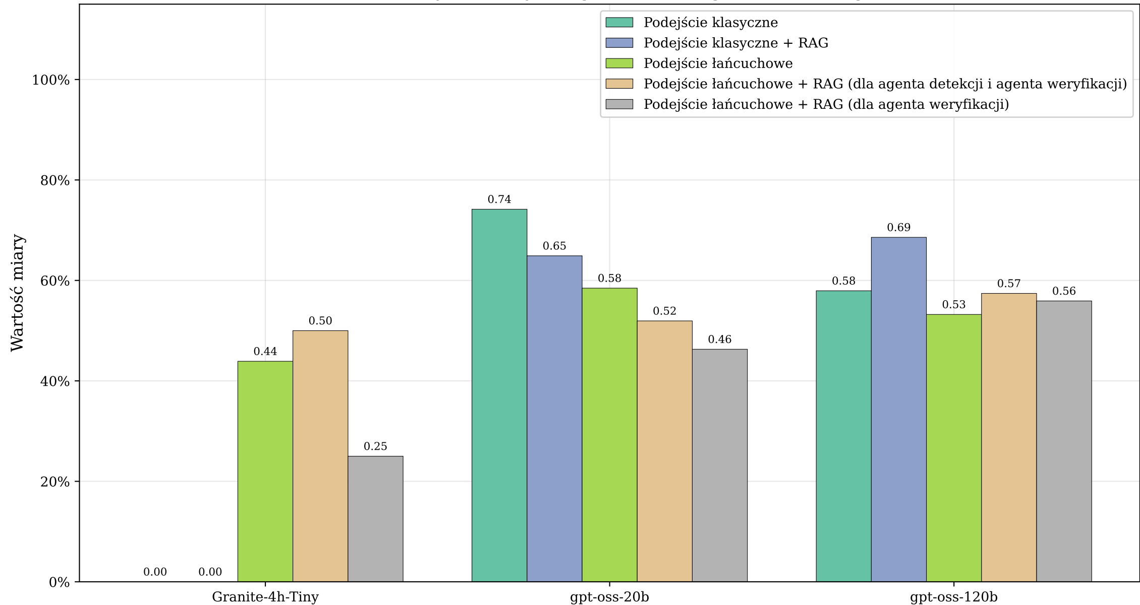
Porównanie miary precyzja dla wybranych dużych modeli językowych oraz podejścia klasycznego i autorskiego łańcuchowego
