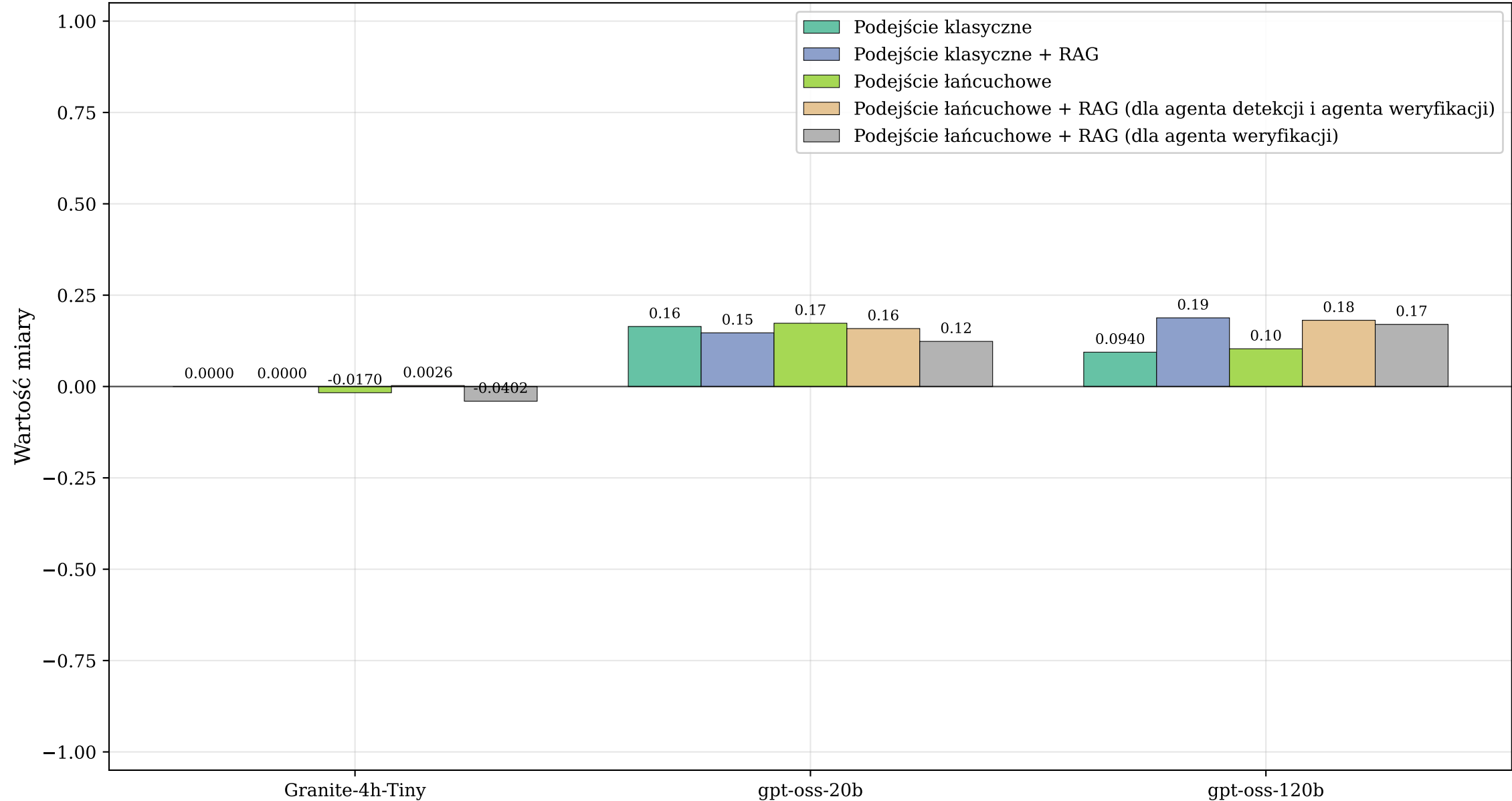
Porównanie miary MCC dla wybranych dużych modeli językowych oraz podejścia klasycznego i autorskiego łańcuchowego
