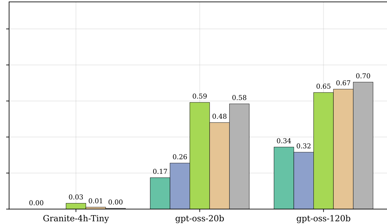
Porównanie miary F2 dla wybranych dużych modeli językowych oraz podejścia klasycznego i autorskiego łańcuchowego
