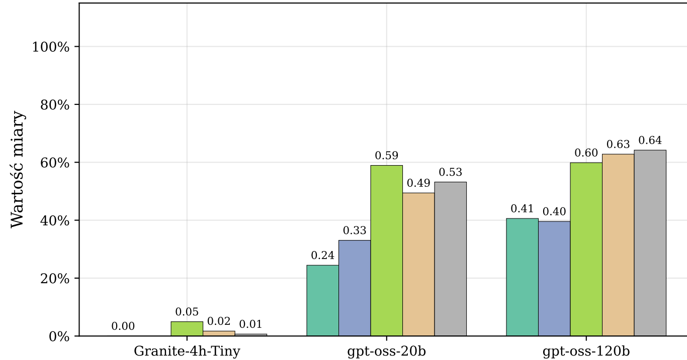
Porównanie miary F1 dla wybranych dużych modeli językowych oraz podejścia klasycznego i autorskiego łańcuchowego
