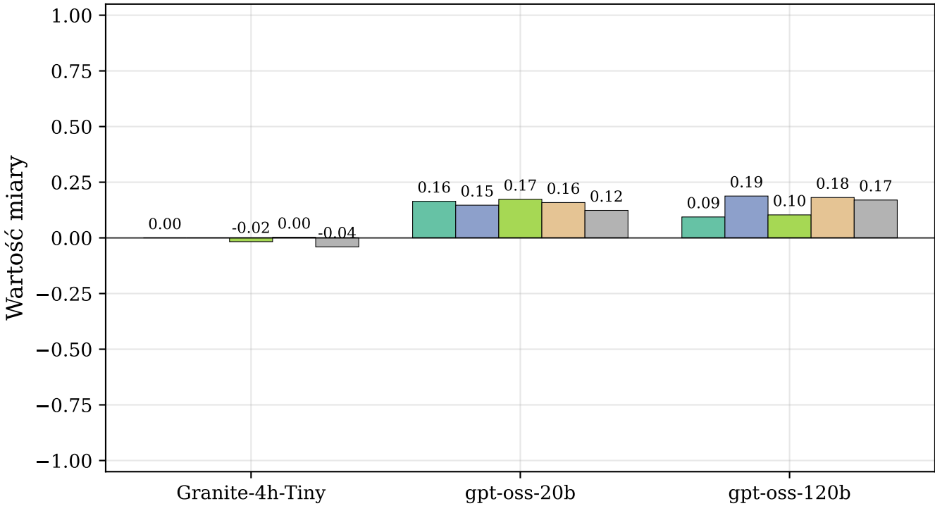
Porównanie miary MCC dla wybranych dużych modeli językowych oraz podejścia klasycznego i autorskiego łańcuchowego
