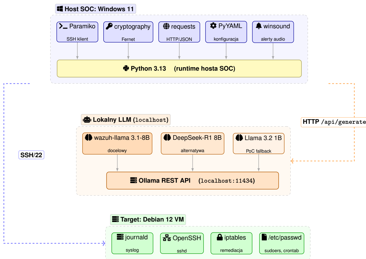
Rys. 3.1. Stos technologiczny SOC AI PoC w podziale na trzy strefy: host Windows (orkiestратор + biblioteki), lokalny LLM (Ollama z trzema modelami) oraz target Debian (komponenty systemowe). Strzałki pokazują dwa kanały komunikacji: SSH (host → VM) i HTTP (host → Ollama).
