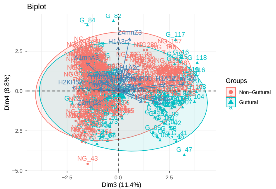
7.4.4.1.3 PCA Biplot 3:4
