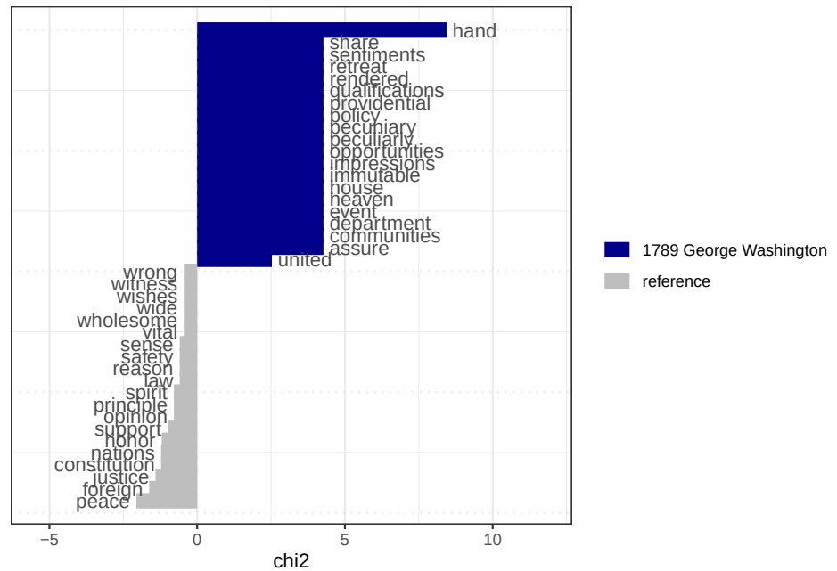
6.4.5.3.2 Plotting
