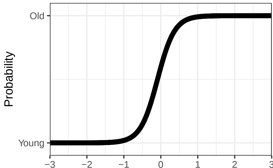
3.4.2.4.4.2 z-scores
