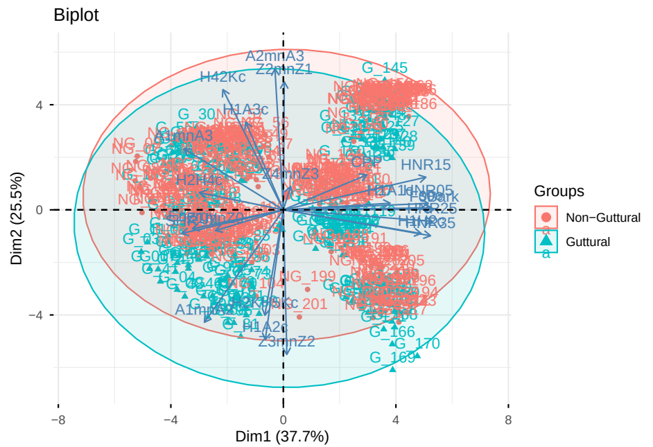
7.4.4.1.2 PCA Biplot 1:2
