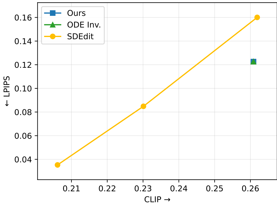
Stable Diffusion 3
