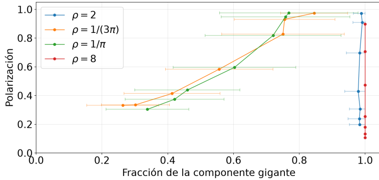
Figura 17: Polarización media \langle v_a \rangle en función de la fracción media del cluster más grande \langle S \rangle (barras de error en ambos ejes), modelo de votante, para \rho = 2, 8, 1/\pi, 1/(3\pi) y \eta \in \{0.05, 0.4, 1\} . 30000 pasos.
