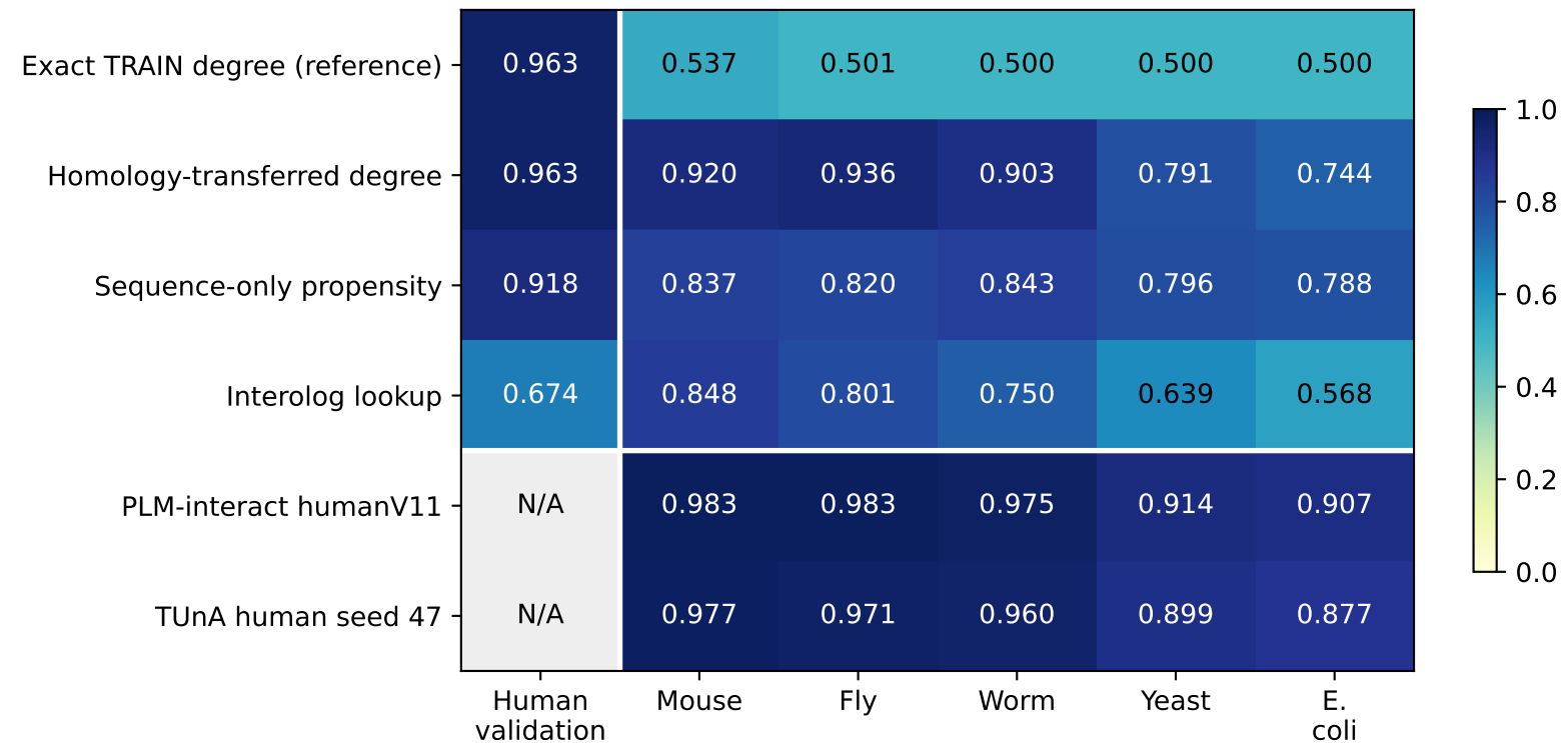
AUROC
