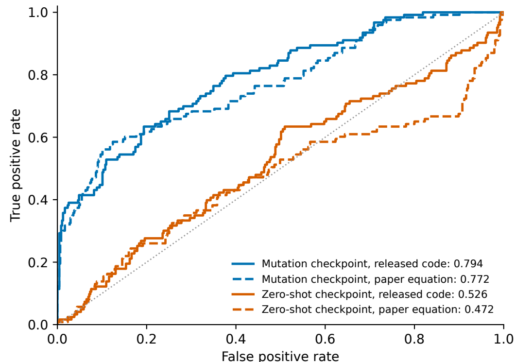
AUROC
