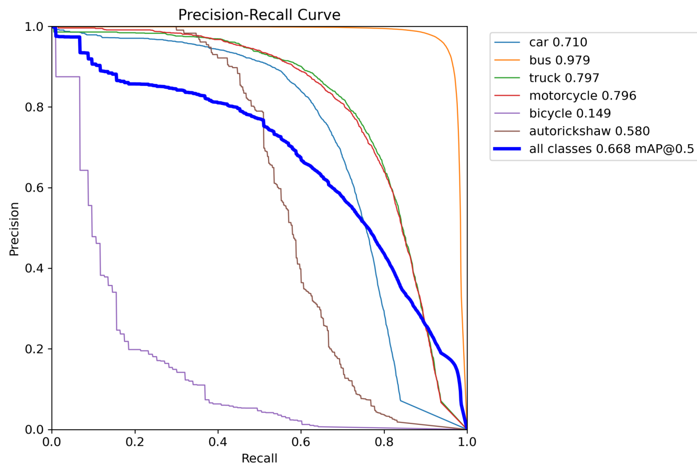
YOLOv12n
