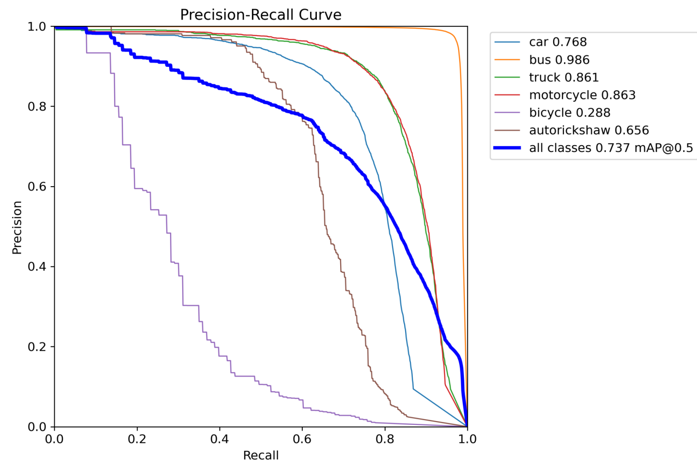
YOLOv12s
