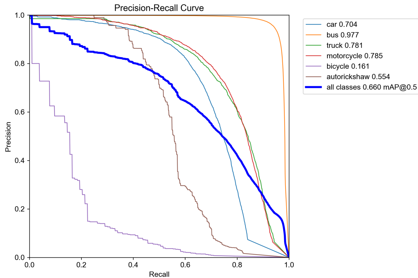
YOLOv11n
