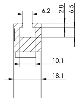
导轨截面尺寸
