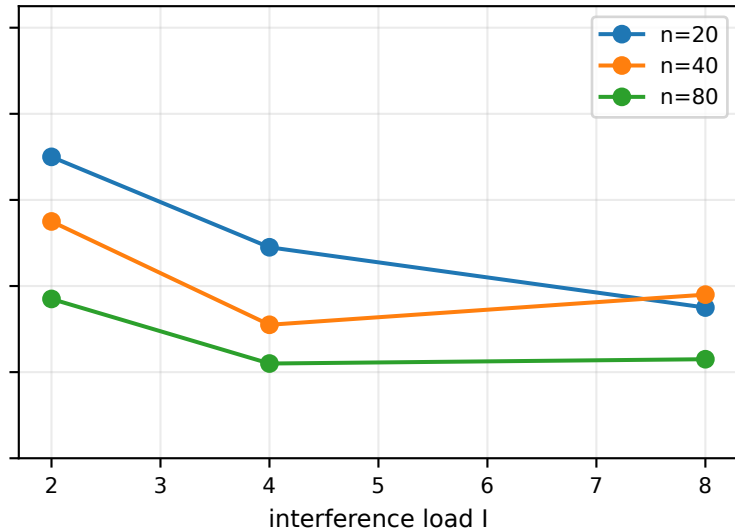
LLAMA
