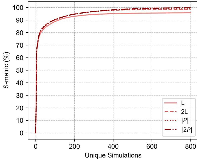
\varepsilon -MOEA
