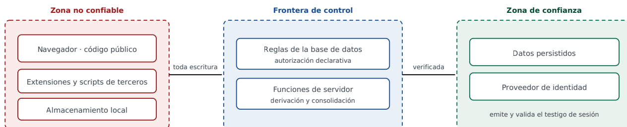
Figura 20.1 — Zonas de confianza y fronteras. Todo lo que está a la izquierda de la frontera de control es territorio del adversario potencial.
