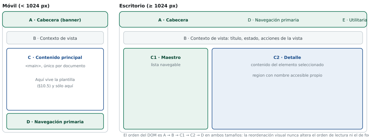
Figura 10.1 — Anatomía del armazón de la aplicación en los dos modos de disposición. Las letras identifican regiones, no componentes: el mismo componente puede ocupar regiones distintas según la plantilla.
