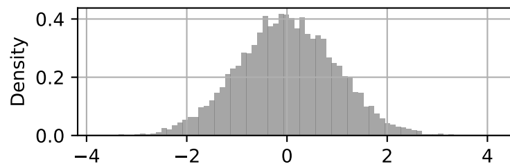
Prior: beta1
