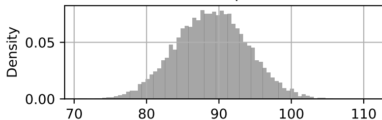
Prior: beta1
