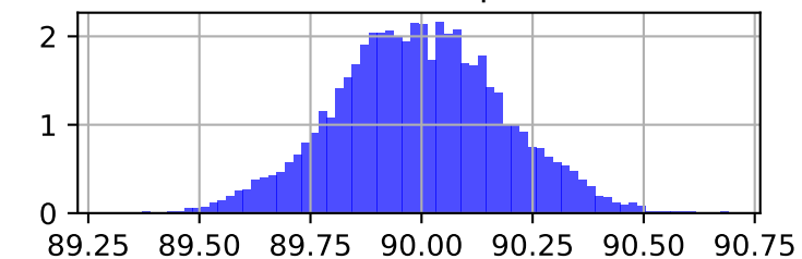
Posterior: alpha2
