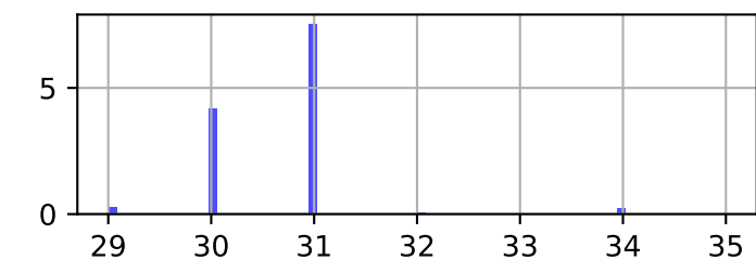
Posterior: tau
