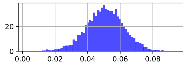
Posterior: beta1
