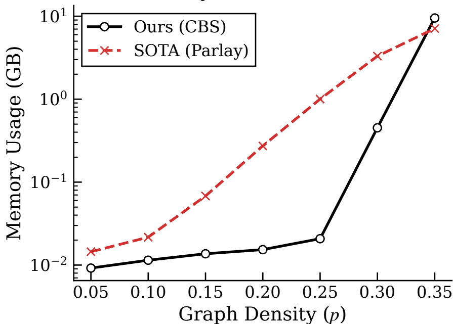
Memory ( N=1000, r=4, s=8 )
