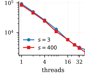
web-it-2004
