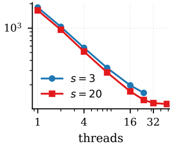
web-Google
