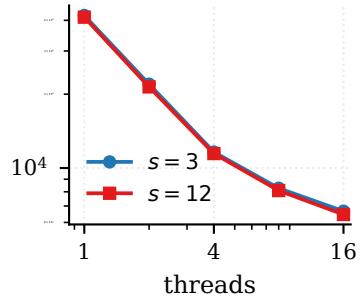
twitter
