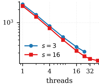
com-youtube
