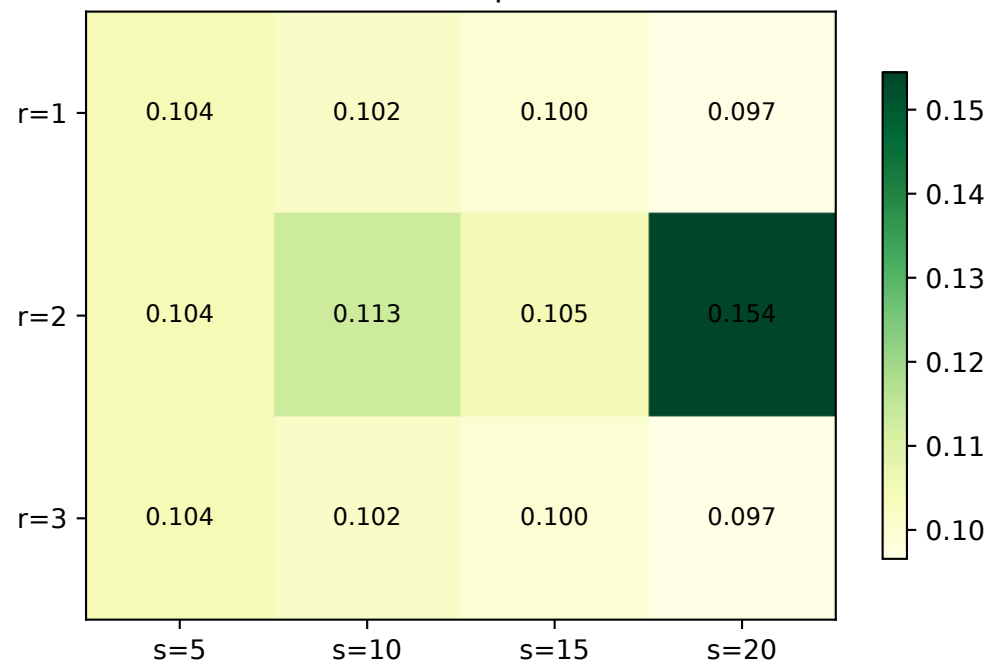
Mean best-F1 top-10 comm.
