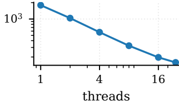
web-Google
