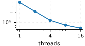
twitter
