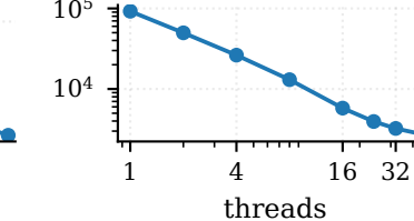
web-it-2004
