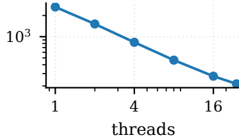
com-youtube
