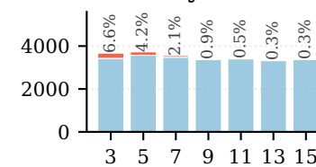
com-youtube
