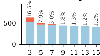
com-dblp
