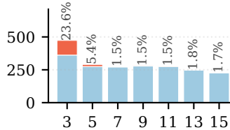
com-amazon
