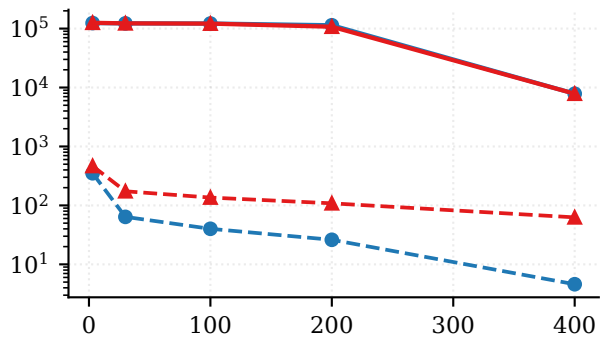
web-it-2004
