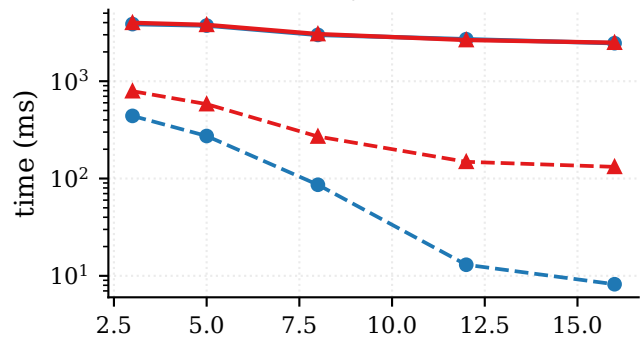
com-youtube
