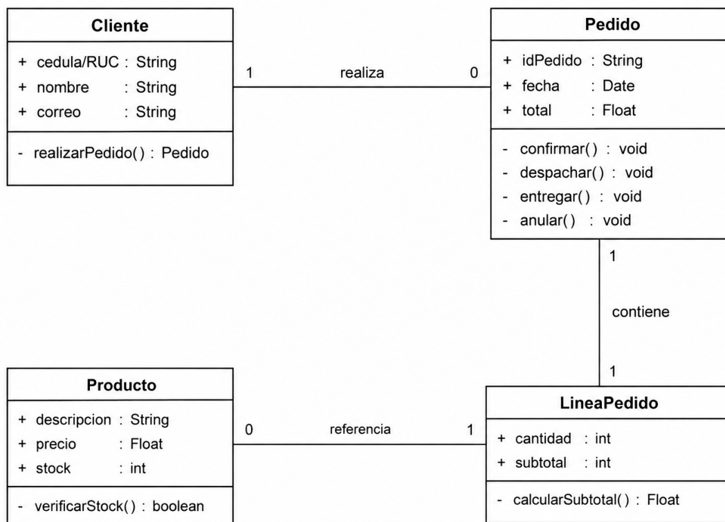
Figura 1: Diagrama de clases UML — Sistema de Gestión de Pedidos
