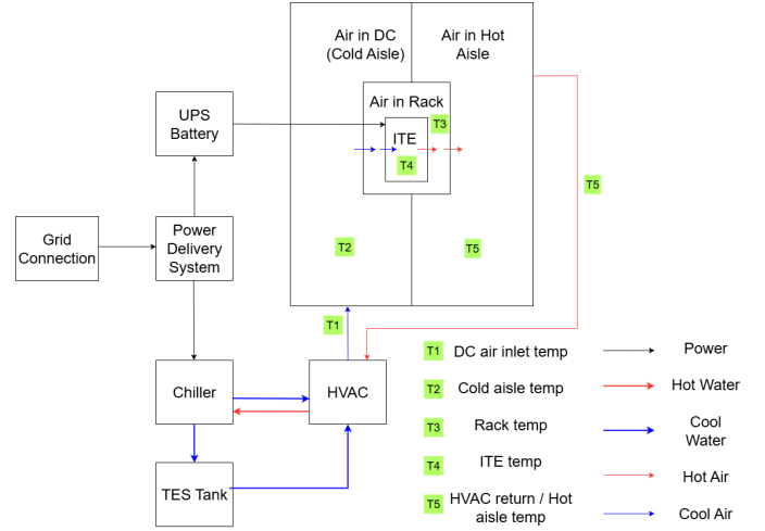
Fig. 1. DC Layout
