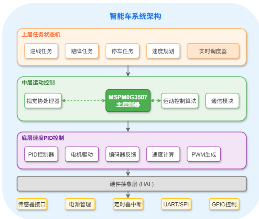
图 1 系统整体流程图
